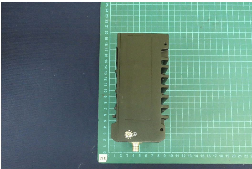
(47) EUT Photo
