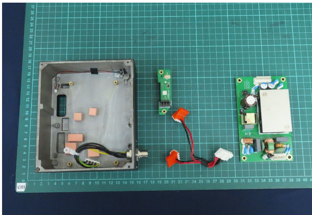
(54) EUT Photo
