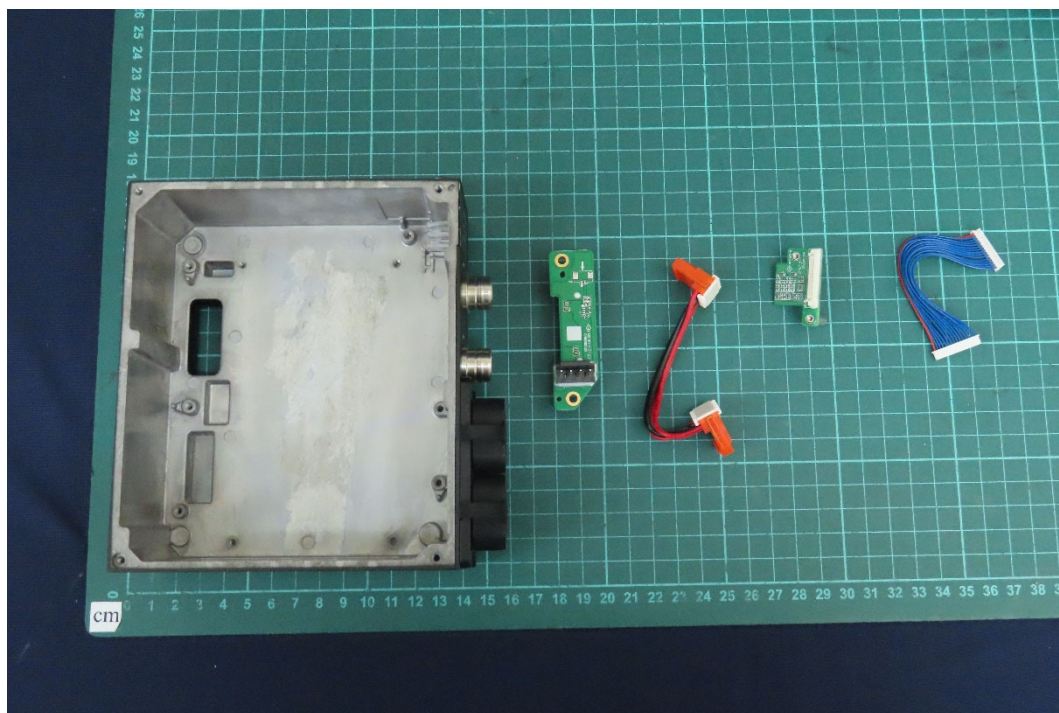
(41) EUT Photo
