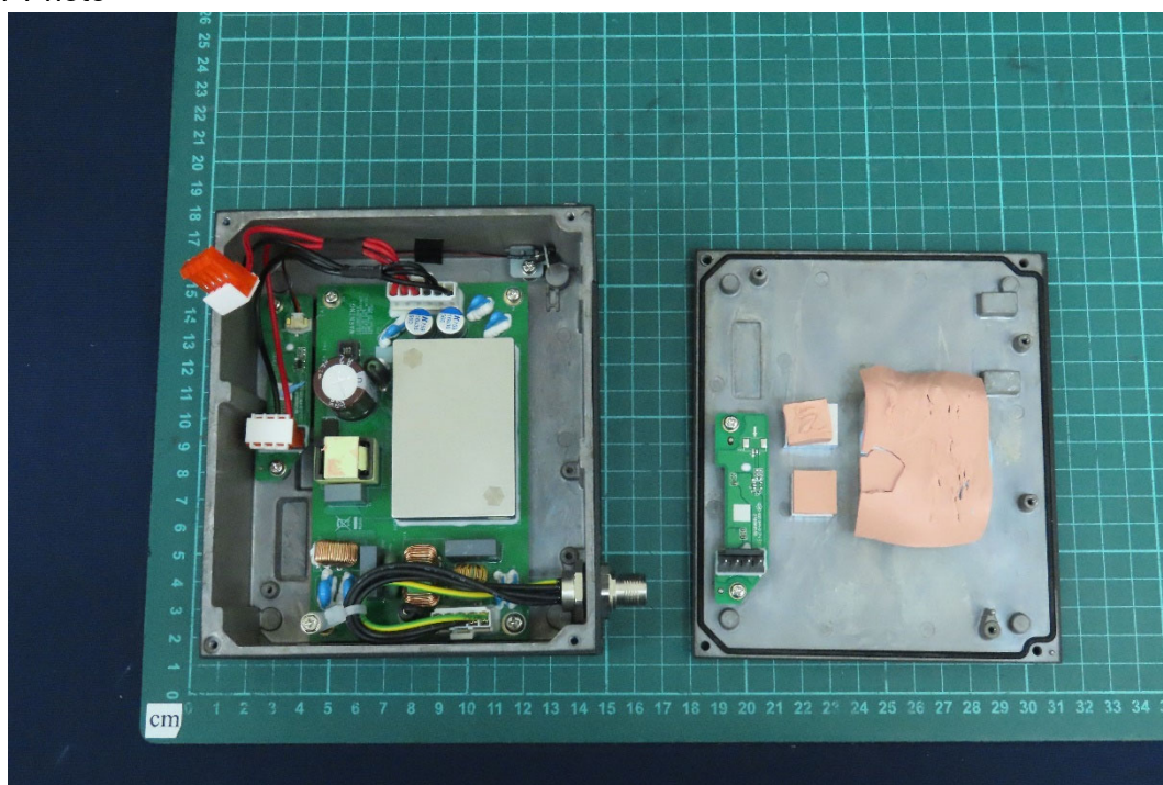
(48) EUT Photo
