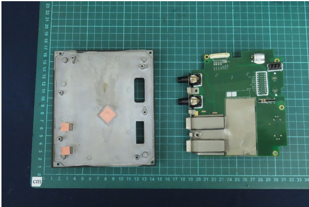
(33) EUT Photo
