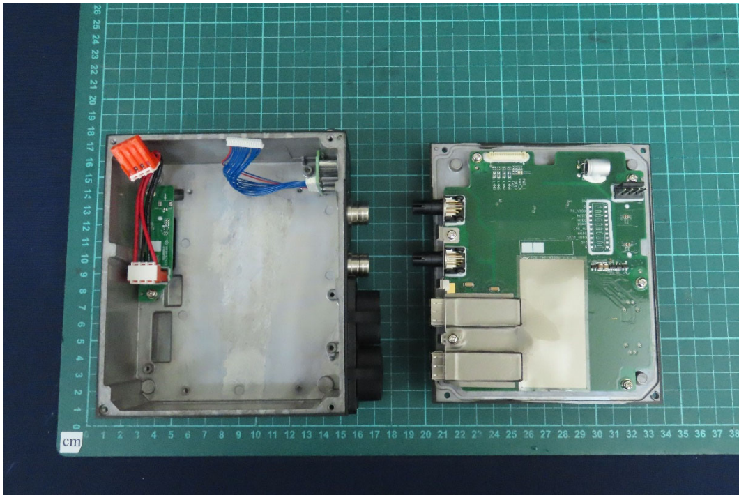
(31) EUT Photo
