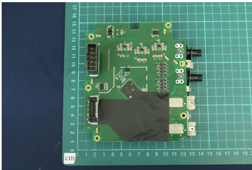
(37) EUT Photo
