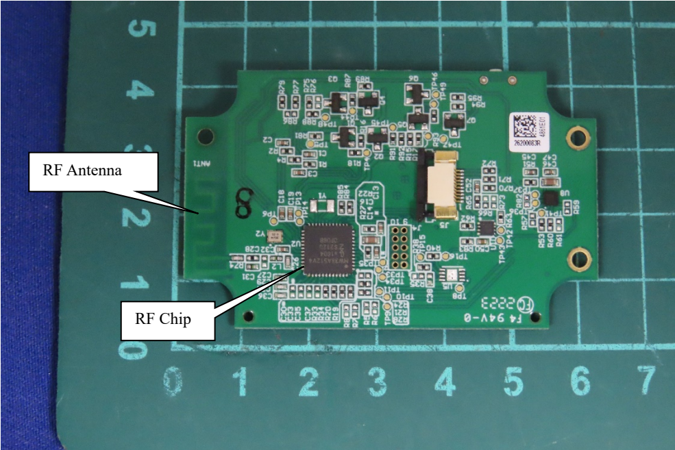
(17) EUT Photo
