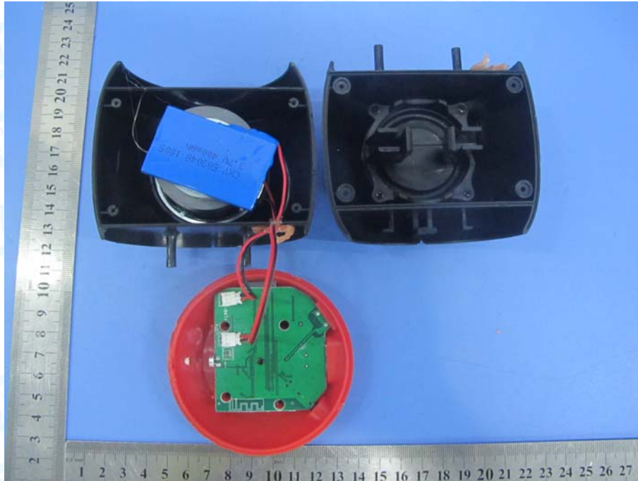
Photo 8 Battery Parameter
