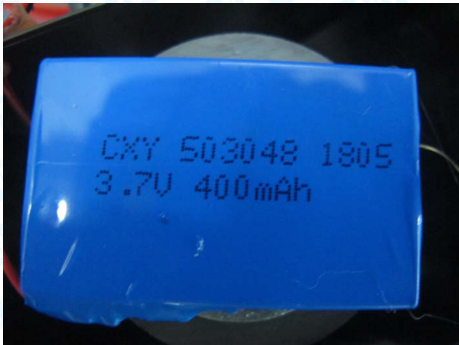
Photo 8 Battery Parameter
