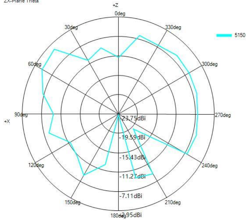
ZX-Plane Theta
