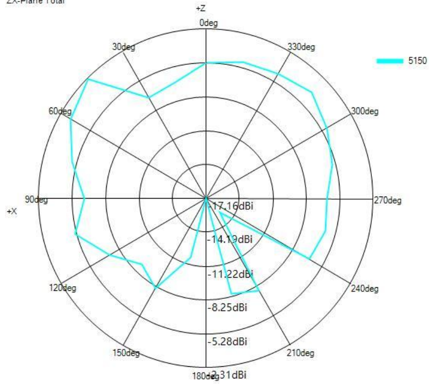
ZX-Plane Total
