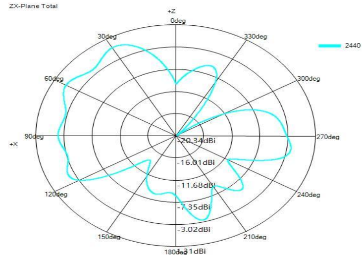
ZX-Plane Total
