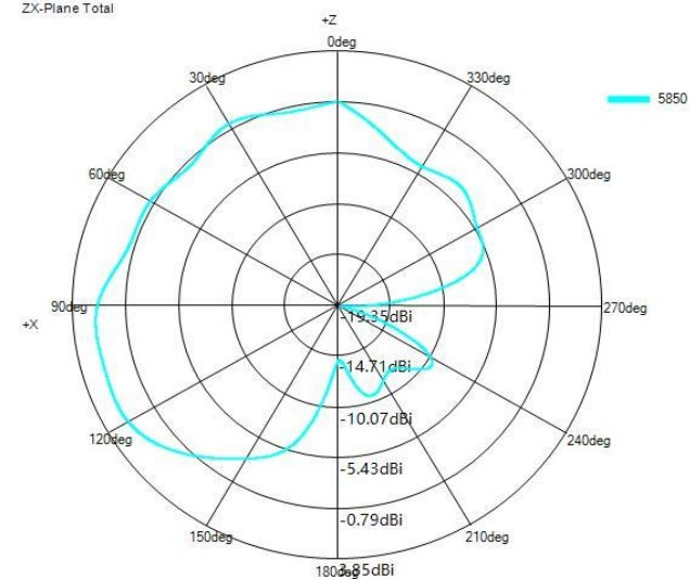
ZX-Plane Total
