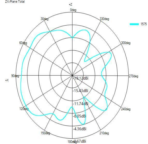
ZX-Plane Total
