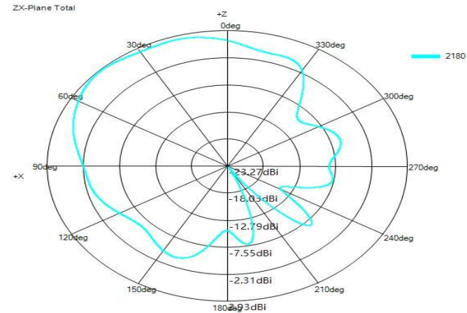
ZX-Plane Total
