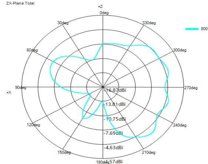
ZX-Plane Total
