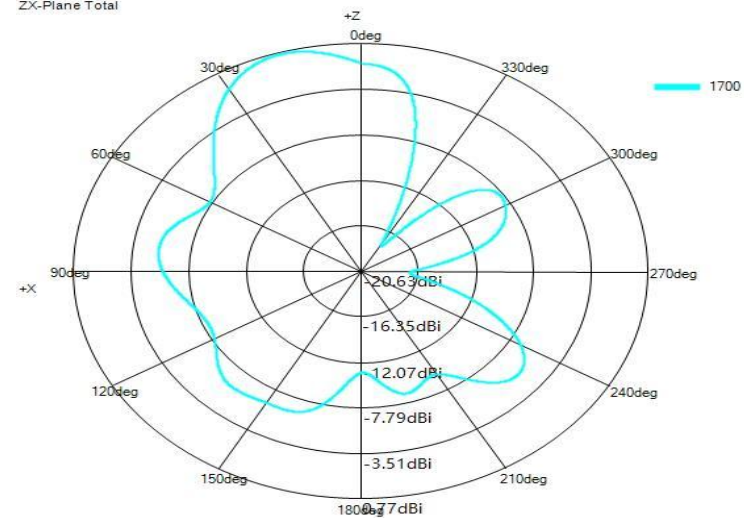
ZX-Plane Total
