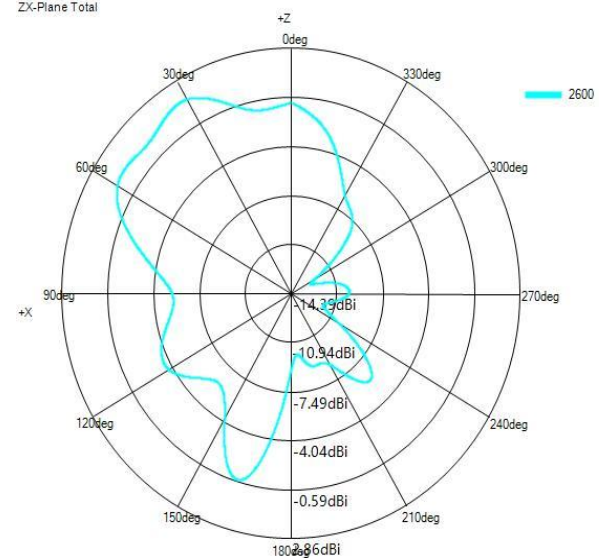
ZX-Plane Total
