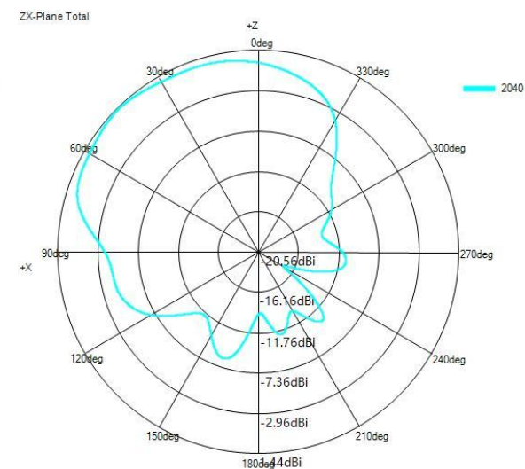
ZX-Plane Total
