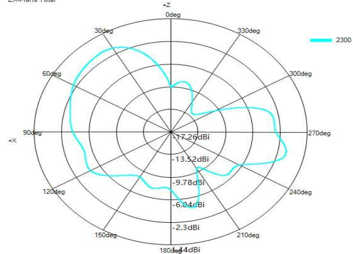
ZX-Plane Total
