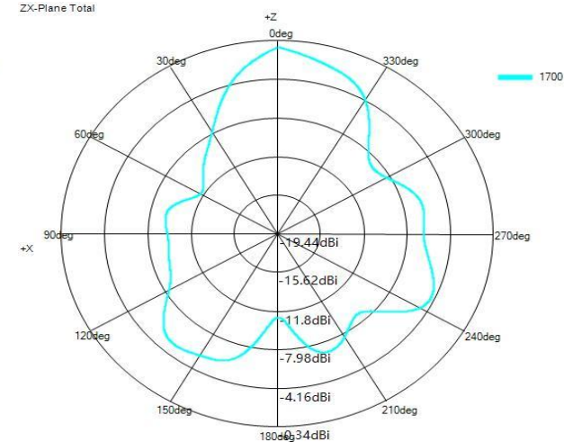
ZX-Plane Total
