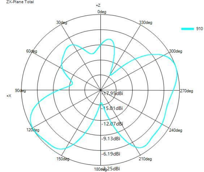
ZX-Plane Total
