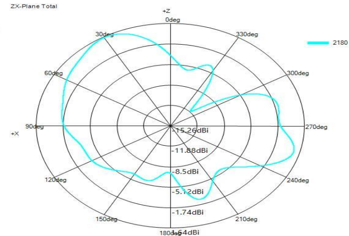
ZX-Plane Total
