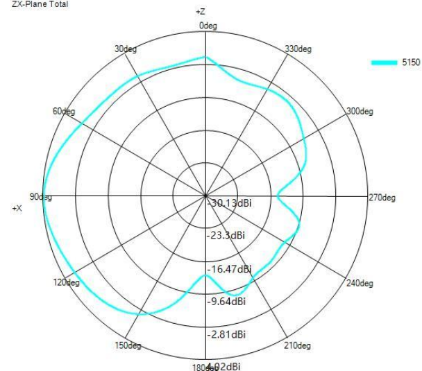
ZX-Plane Total
