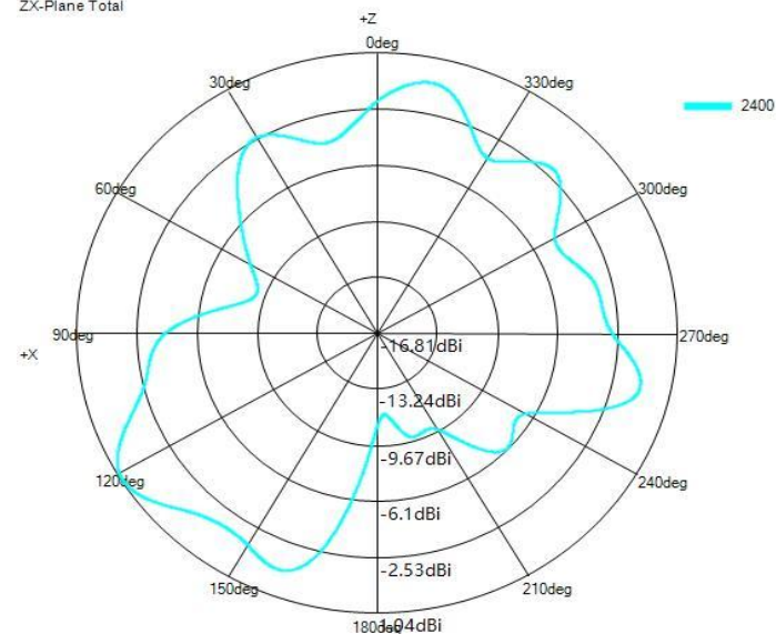
ZX-Plane Total
