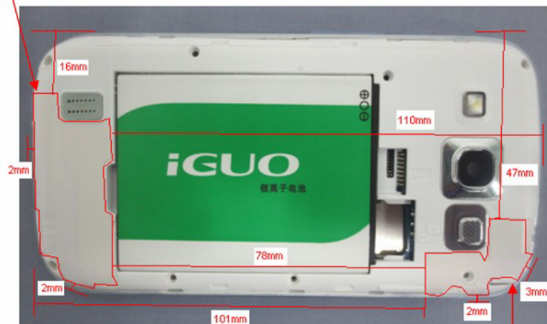
GSM Antenna
