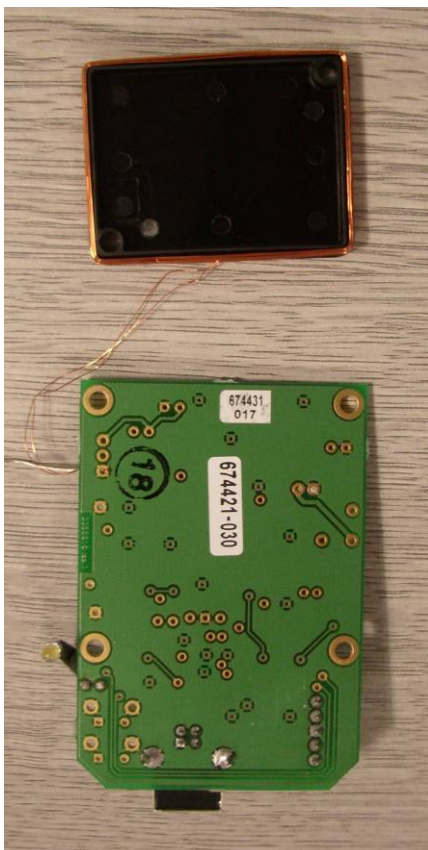
PCB Bottom
