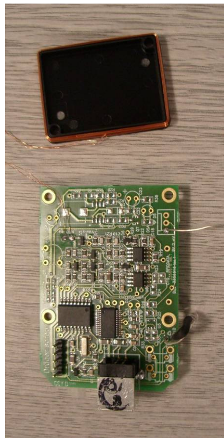
PCB Top
