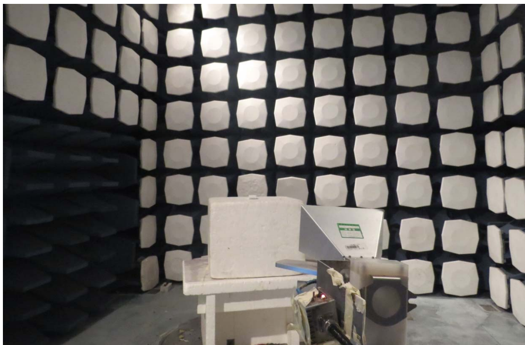
1GHz-18GHz
