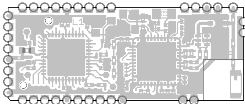
Figure 1: nanoLOC AVR Module - top side
