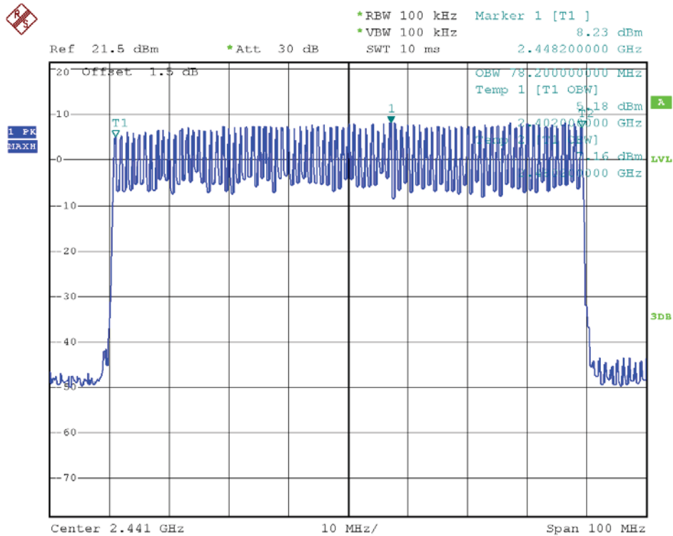
(Plot A:GFSK)
