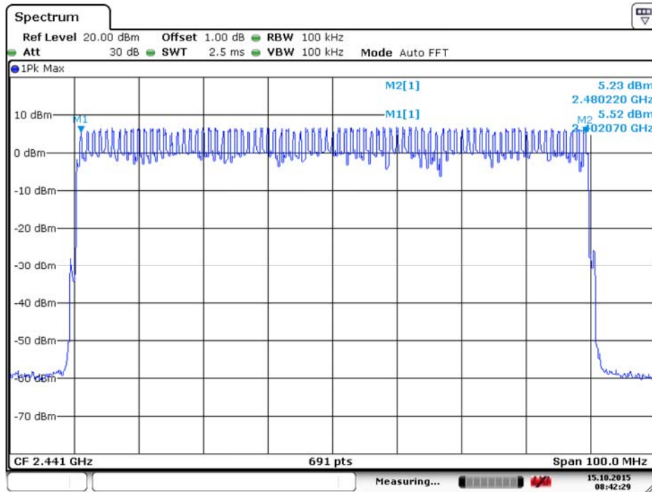
(Plot B: \pi/4 -DQPSK)
