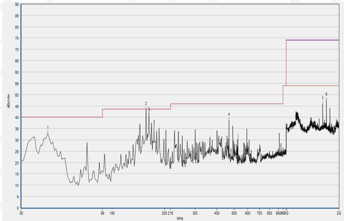
(Plot A: 30MHz – 2GHz, Test Antenna Vertical)
