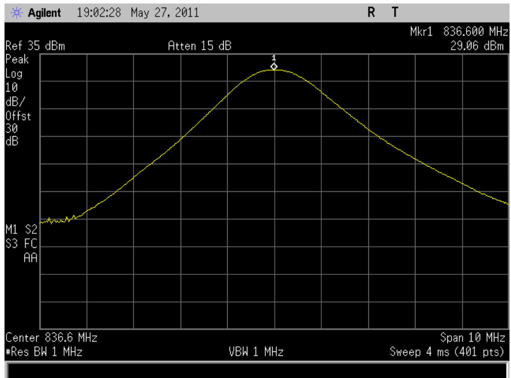
(Plot D: GSM 850MHz Channel = 190)
