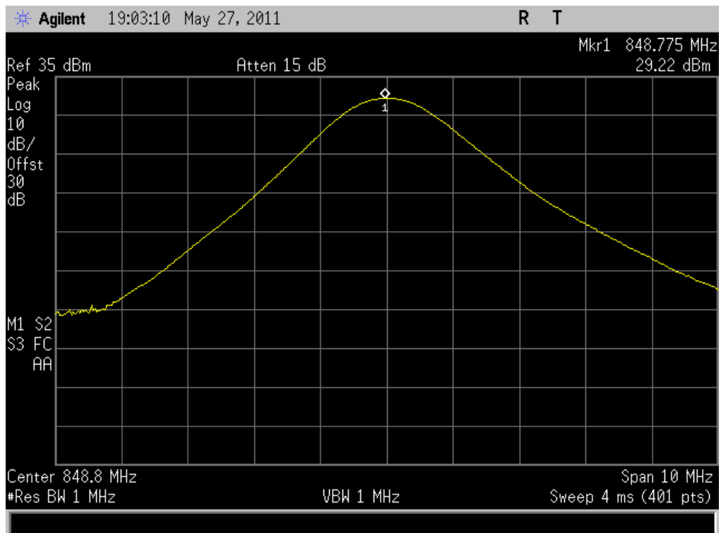
(Plot E: GSM 850MHz Channel = 251)
