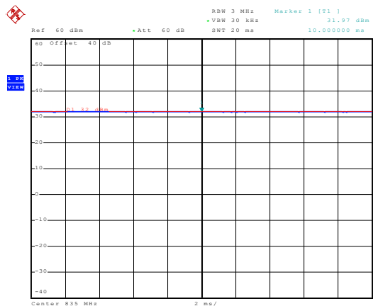
835MHz - CW
