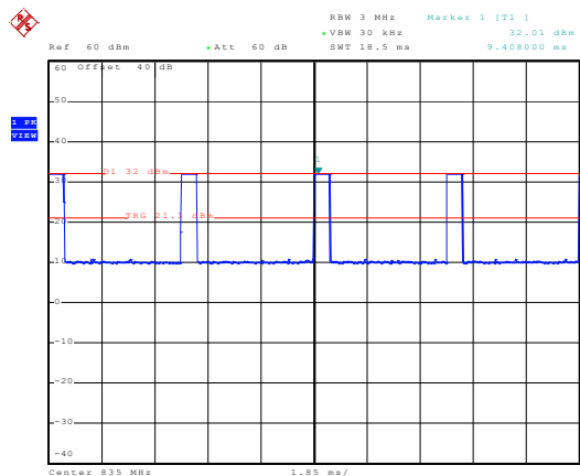
835MHz - GSM
