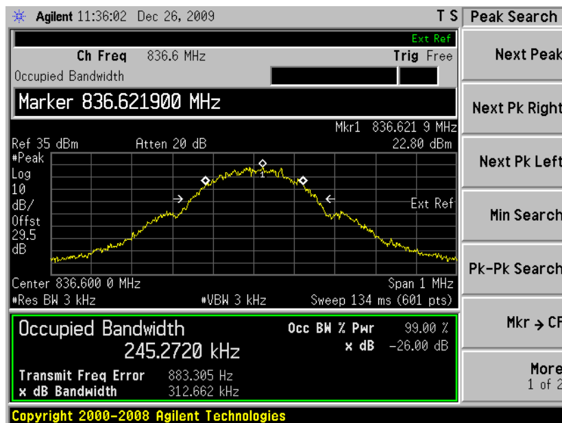
(Plot B: GSM 850MHz Channel = 190)
