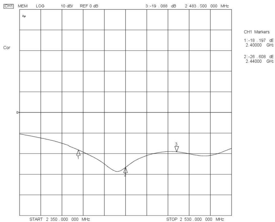
Fig. 1. Return Loss
