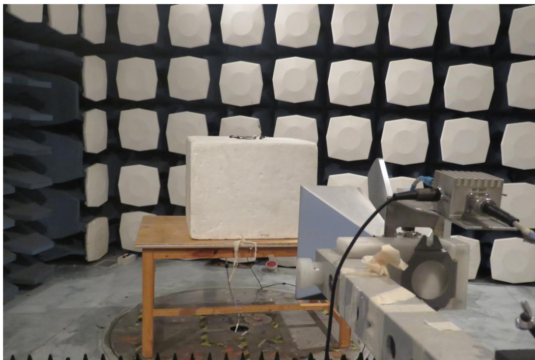
1GHz-18GHz
