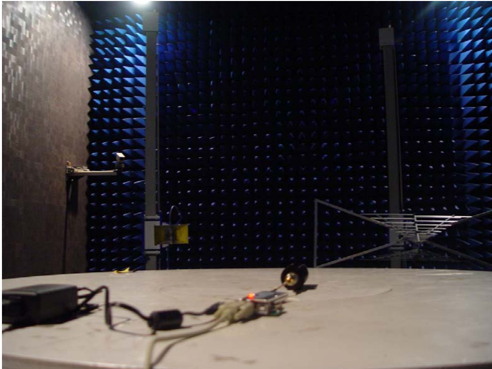
E.R.P. Test Setup
