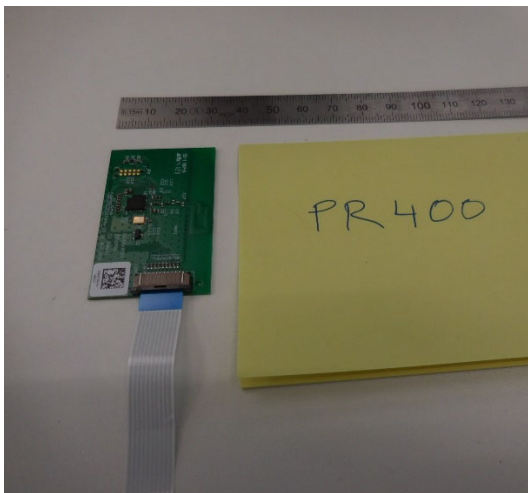
BLE Board
