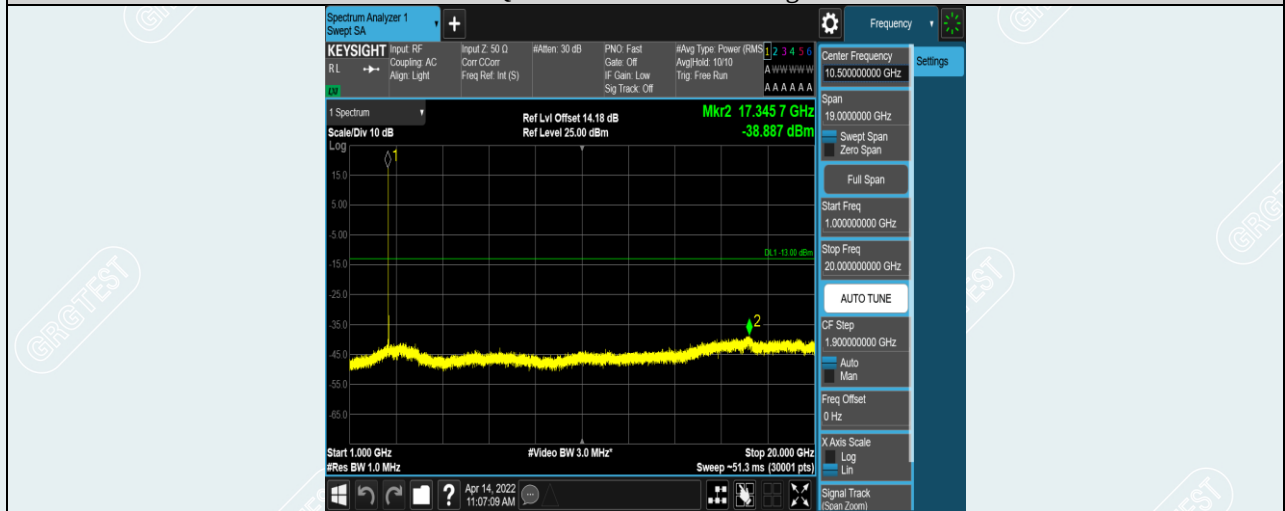
Band38-20MHz-QPSK-37850-1RB#0-Range2:1000~20000MHz
