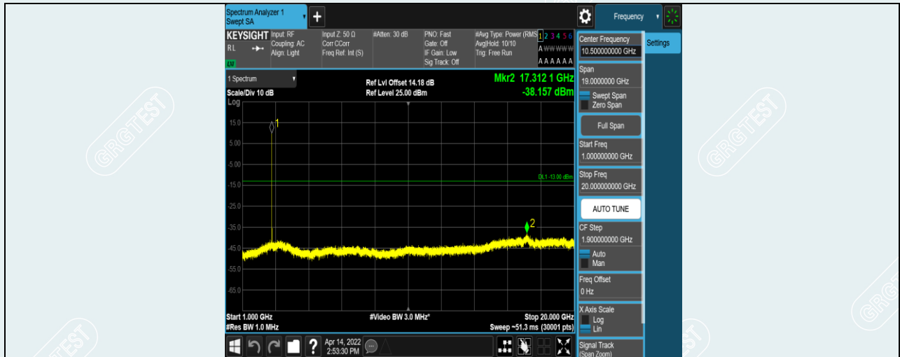
Band41-5MHz-QPSK-41565-1RB#0-Range2:1000~20000MHz
