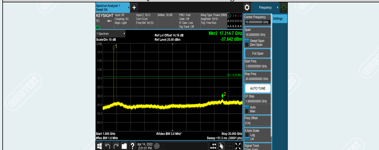
Band41-5MHz-QPSK-39675-1RB#0-Range2:1000~20000MHz
