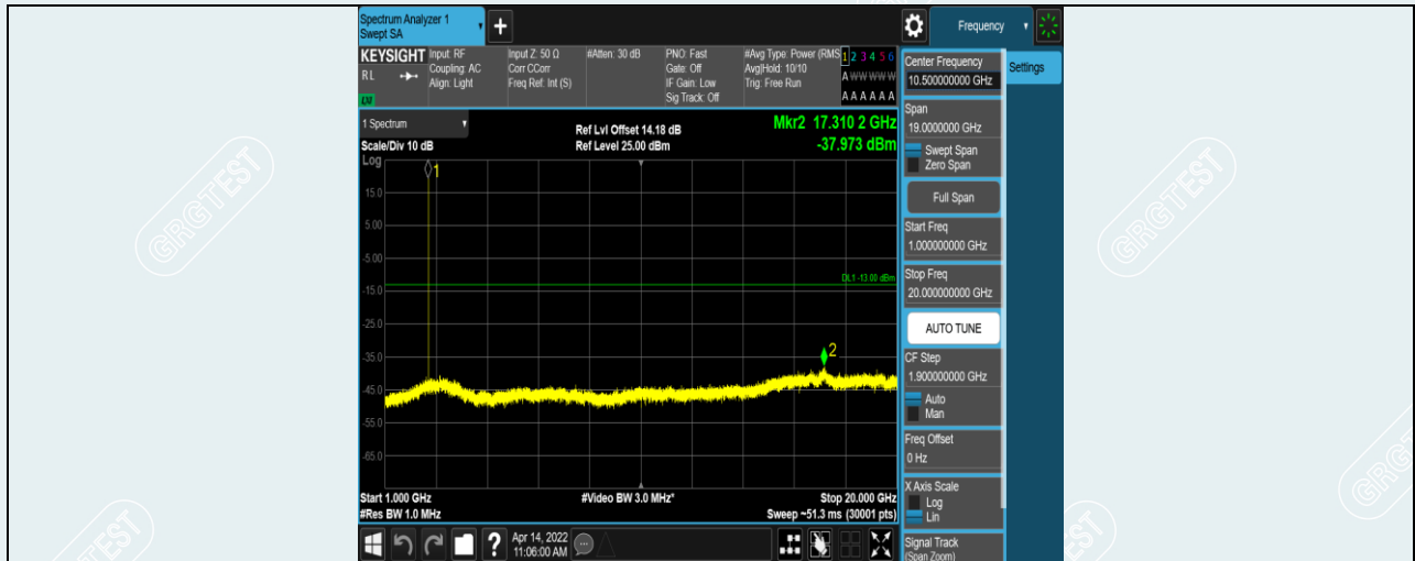
Band38-5MHz-QPSK-38225-1RB#0-Range2:1000~20000MHz
