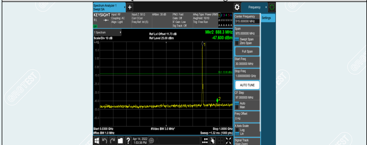
Band13-5MHz-QPSK-23230-1RB#0-Range4:30~1000MHz
