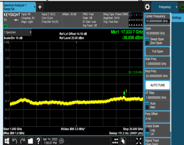
Band13-5MHz-QPSK-23255-1RB#0-Range5:1000~20000MHz
