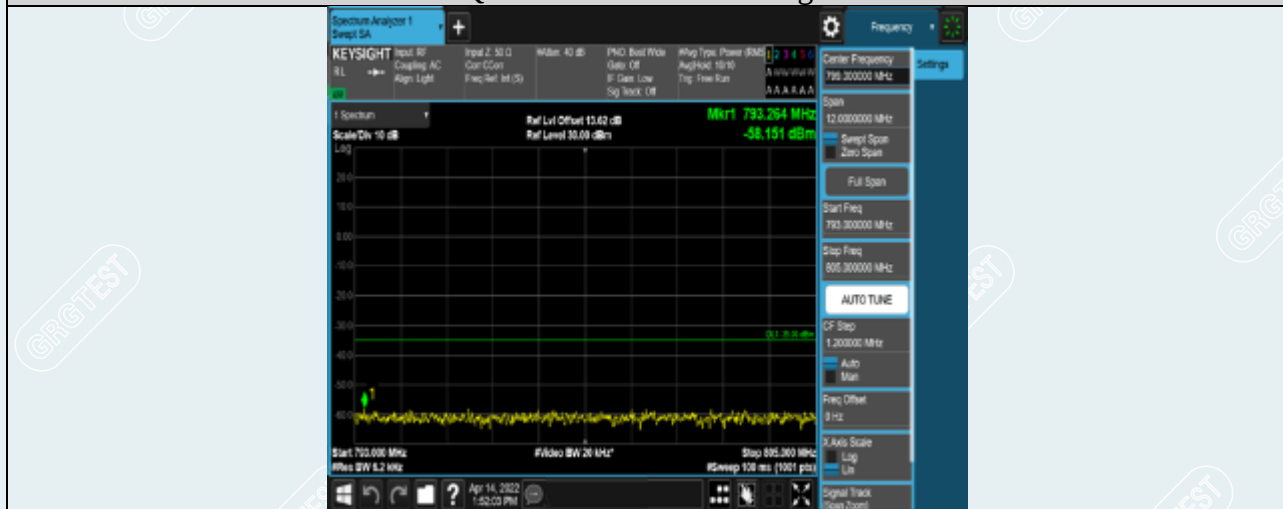
Band13-5MHz-QPSK-23205-1RB#0-Range2:793~805MHz
