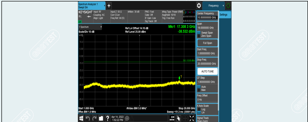
Band13-5MHz-QPSK-23205-1RB#0-Range5:1000~20000MHz
