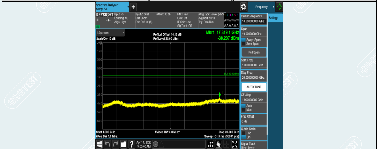
Band12-10MHz-QPSK-23130-1RB#0-Range2:1000~20000MHz
