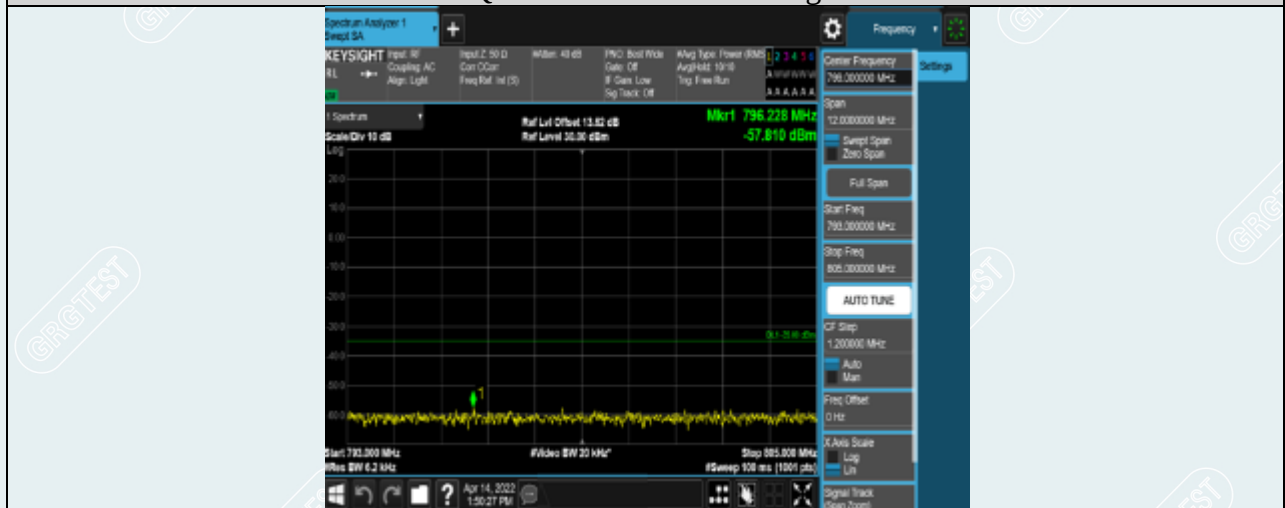
Band13-10MHz-QPSK-23230-1RB#0-Range2:793~805MHz
