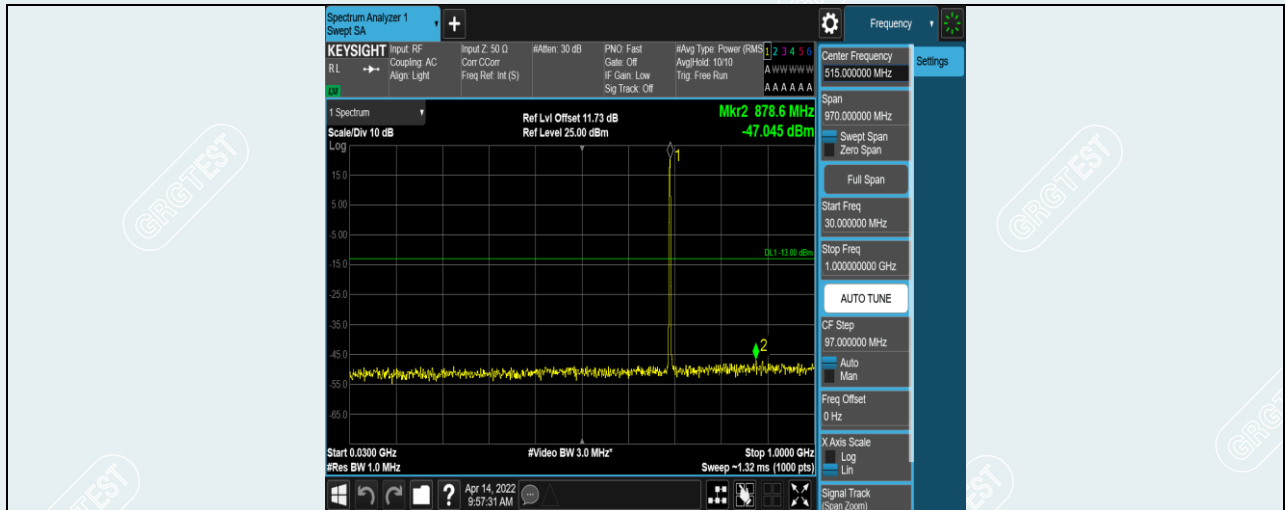
Band12-1.4MHz-QPSK-23017-1RB#0-Range1:30~1000MHz
