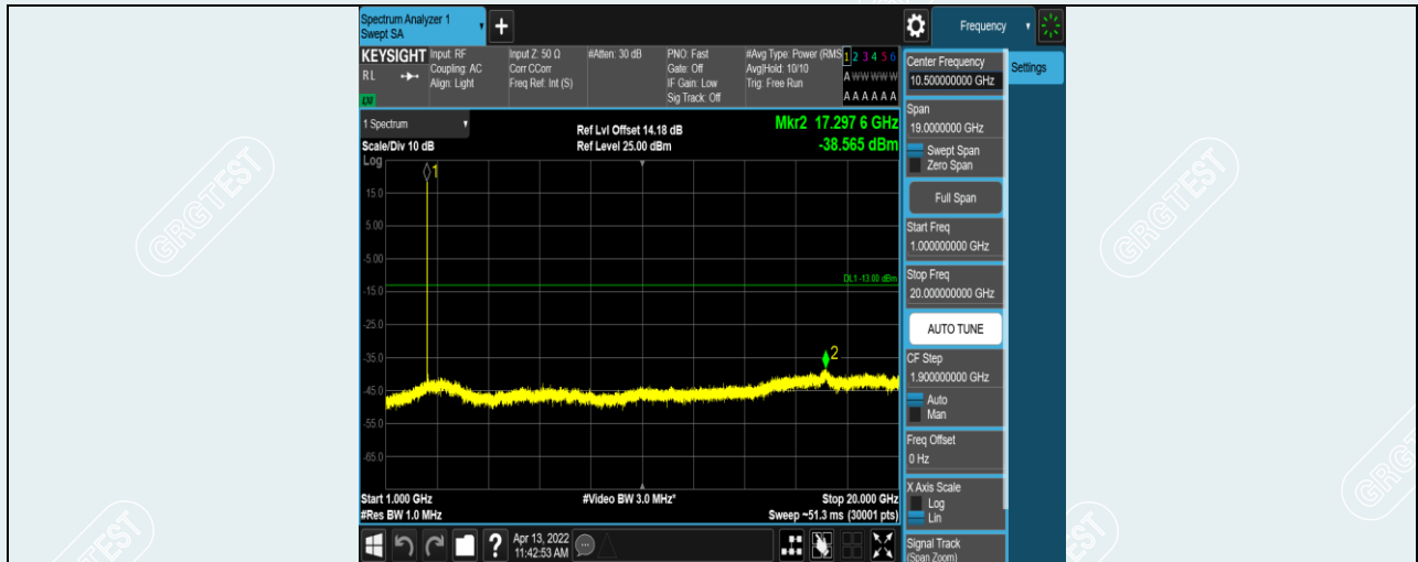
Band7-20MHz-QPSK-21100-1RB#0-Range2:1000~20000MHz
