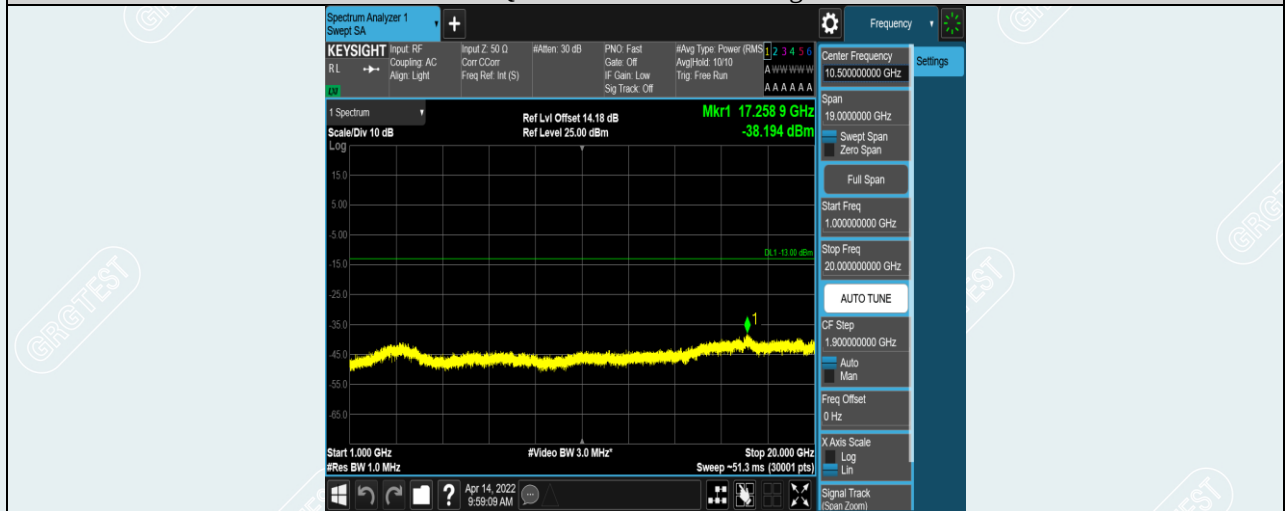
Band12-1.4MHz-QPSK-23173-1RB#0-Range2:1000~20000MHz
