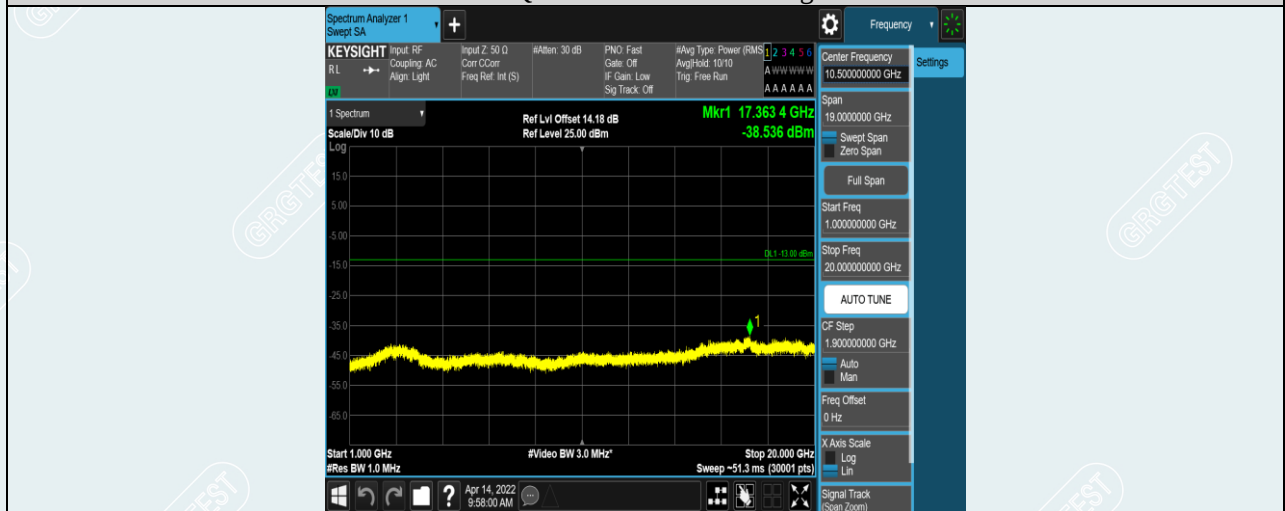
Band12-1.4MHz-16QAM-23017-1RB#0-Range2:1000~20000MHz
