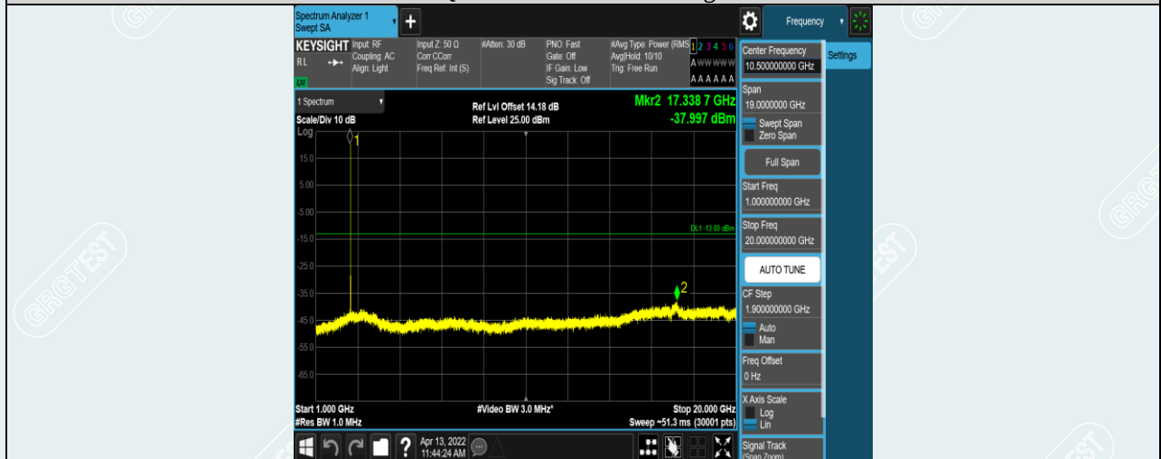
Band7-20MHz-QPSK-21350-1RB#0-Range2:1000~20000MHz
