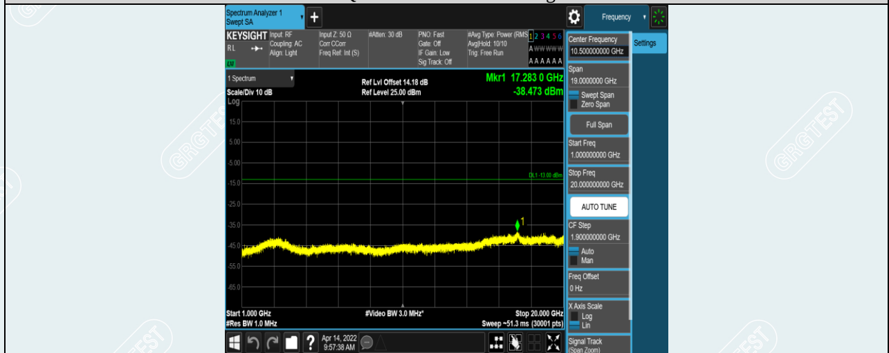
Band12-1.4MHz-QPSK-23017-1RB#0-Range2:1000~20000MHz
