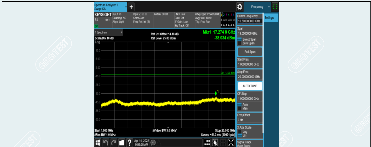
Band12-3MHz-QPSK-23095-1RB#0-Range2:1000~20000MHz
