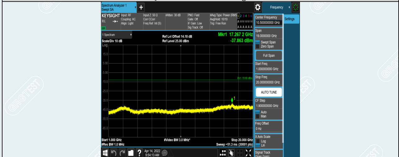
Band12-3MHz-QPSK-23165-1RB#0-Range2:1000~20000MHz
