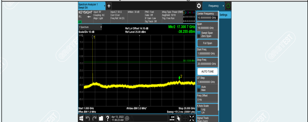
Band7-10MHz-QPSK-20800-1RB#0-Range2:1000~20000MHz
