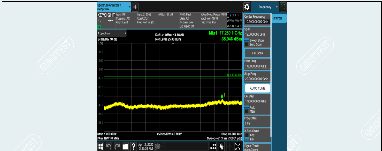
Band5-10MHz-QPSK-20525-1RB#0-Range2:1000~20000MHz
