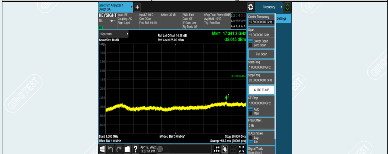
Band5-10MHz-QPSK-20600-1RB#0-Range2:1000~20000MHz
