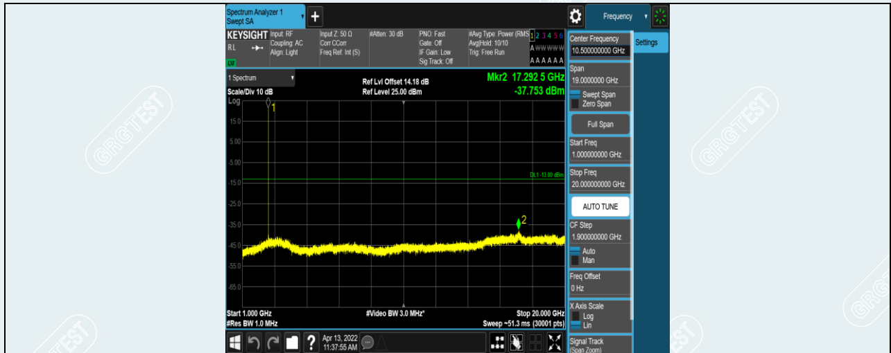
Band7-10MHz-QPSK-21100-1RB#0-Range2:1000~20000MHz
