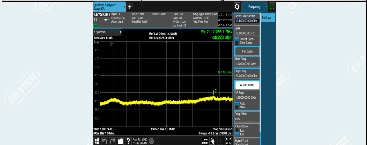
Band7-5MHz-QPSK-21425-1RB#0-Range2:1000~20000MHz
