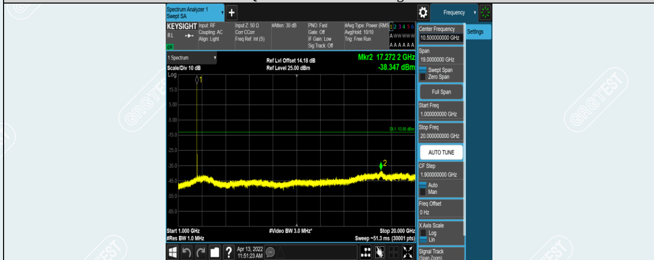
Band7-15MHz-QPSK-20825-1RB#0-Range2:1000~20000MHz
