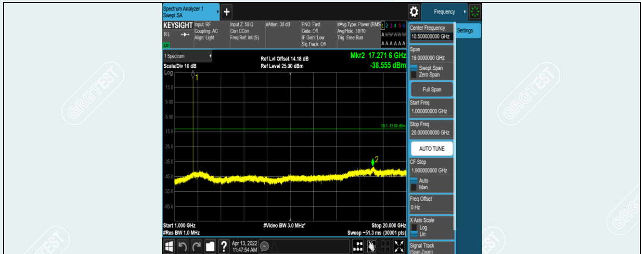
Band7-5MHz-QPSK-21100-1RB#0-Range2:1000~20000MHz
