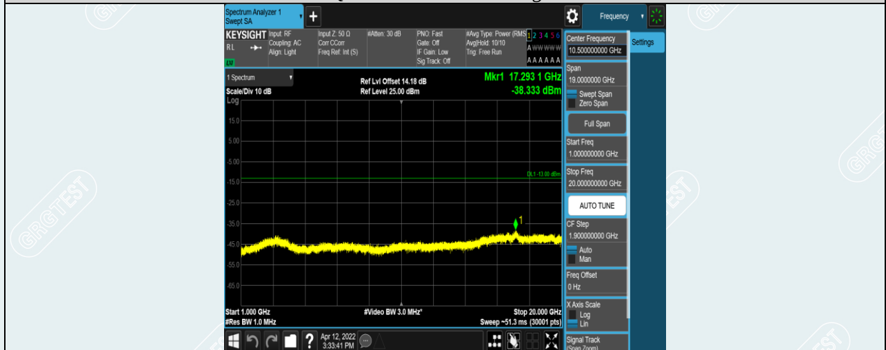
Band5-5MHz-QPSK-20625-1RB#0-Range2:1000~20000MHz
