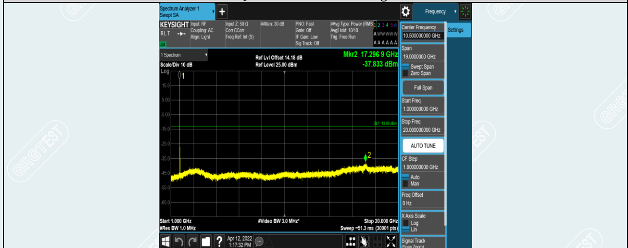
Band4-20MHz-QPSK-20300-1RB#0-Range2:1000~20000MHz
