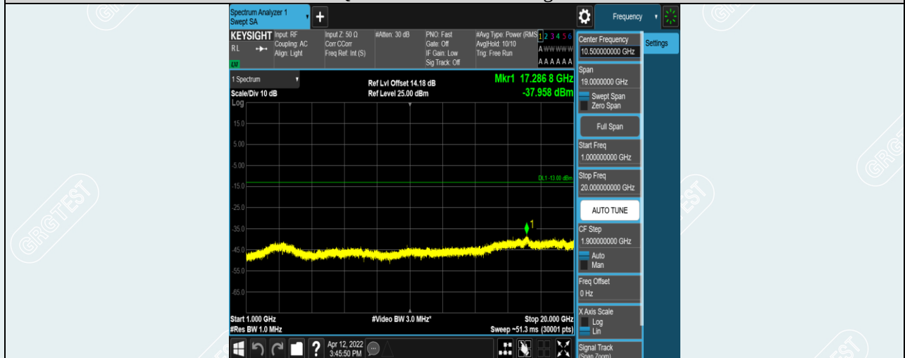
Band5-3MHz-QPSK-20635-1RB#0-Range2:1000~20000MHz
