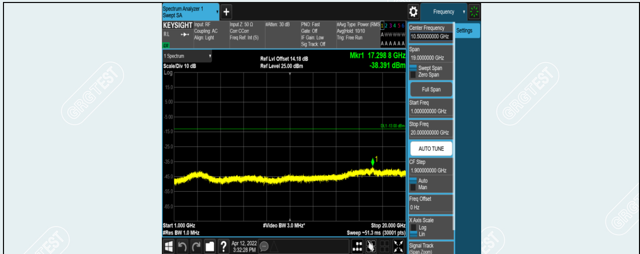
Band5-5MHz-QPSK-20525-1RB#0-Range2:1000~20000MHz
