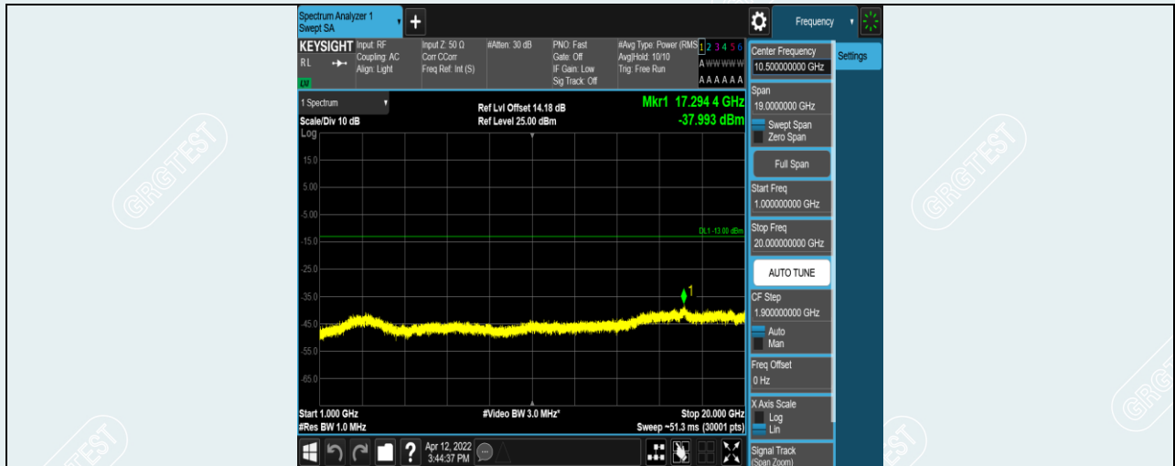
Band5-3MHz-QPSK-20525-1RB#0-Range2:1000~20000MHz
