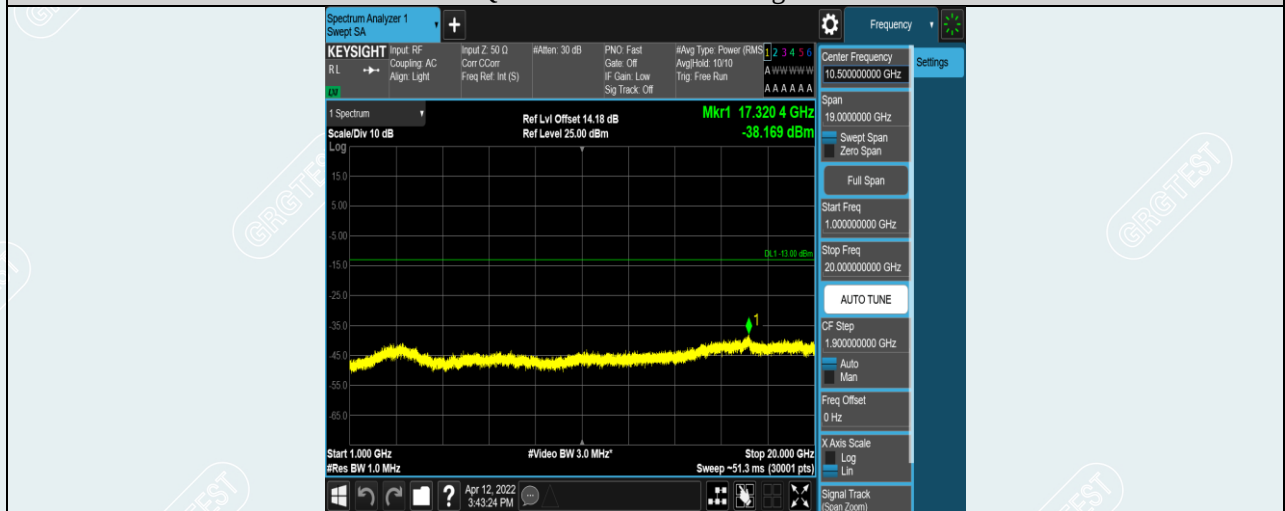
Band5-3MHz-QPSK-20415-1RB#0-Range2:1000~20000MHz
