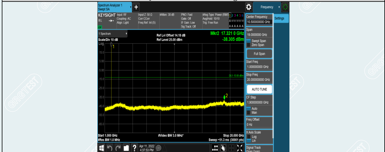
Band2-15MHz-QPSK-19125-1RB#0-Range2:1000~20000MHz
