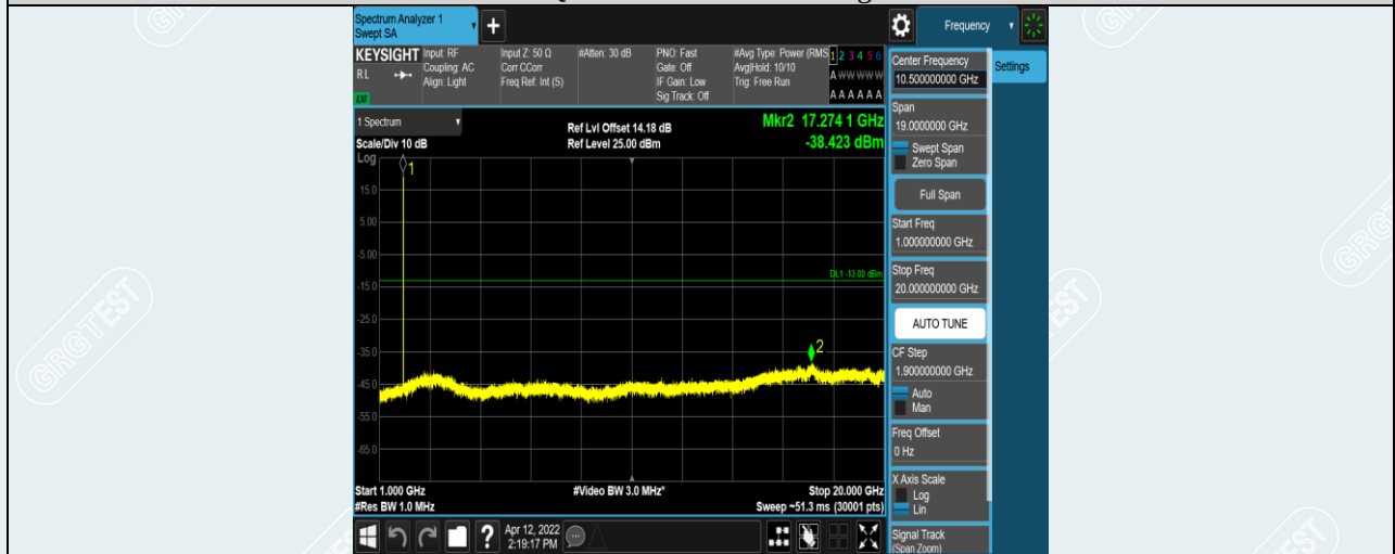
Band2-20MHz-16QAM-19100-1RB#0-Range2:1000~20000MHz
