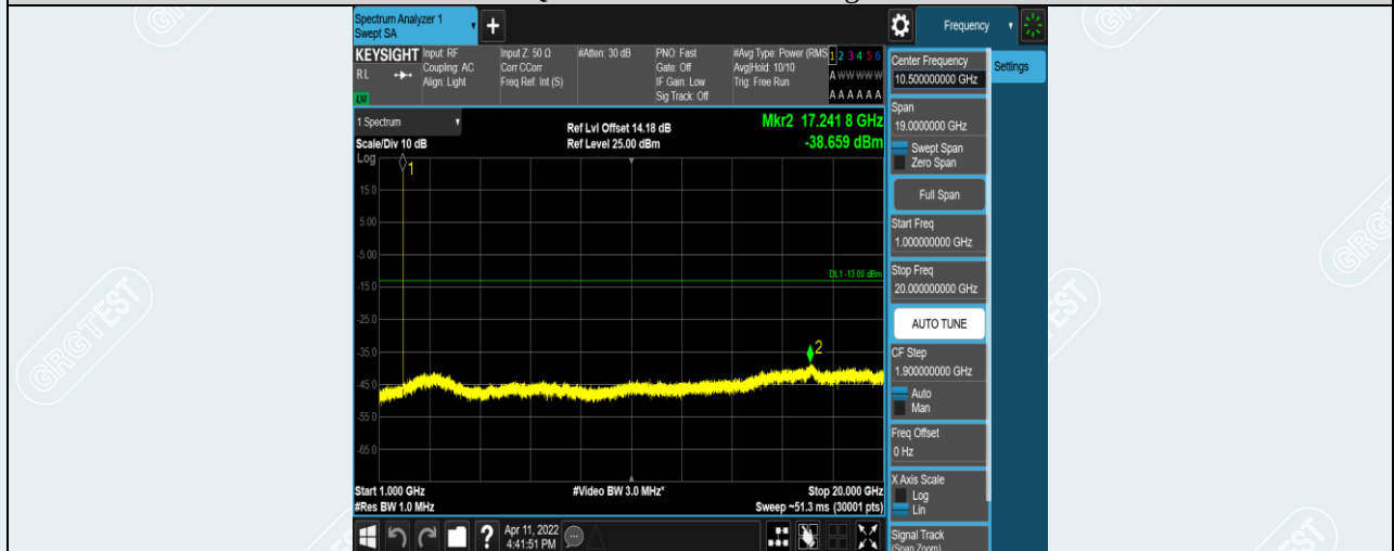
Band2-10MHz-QPSK-19150-1RB#0-Range2:1000~20000MHz
