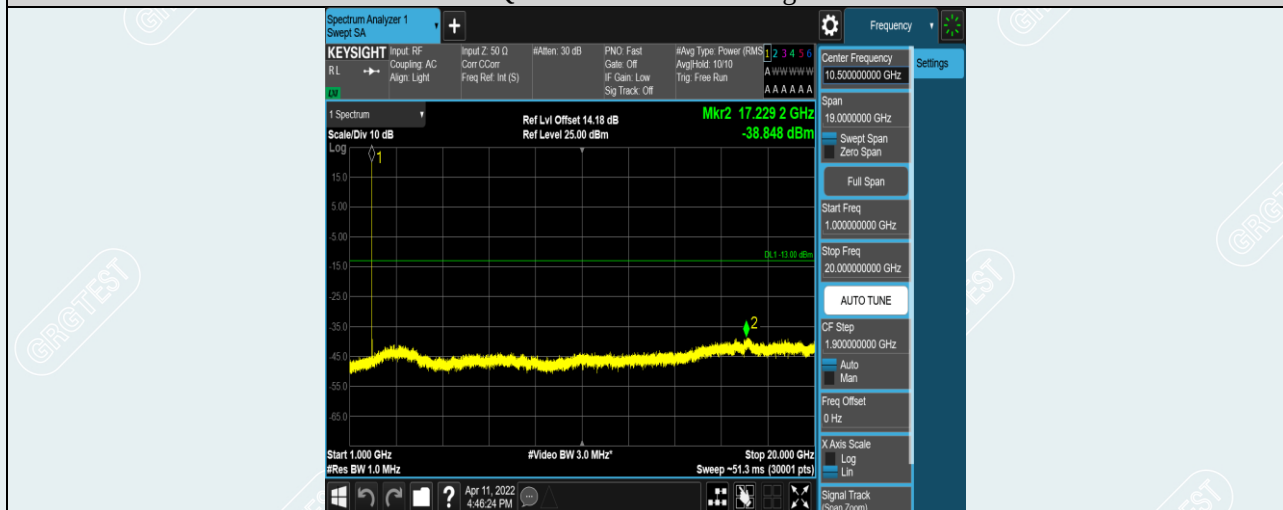
Band2-5MHz-16QAM-19175-1RB#0-Range2:1000~20000MHz
