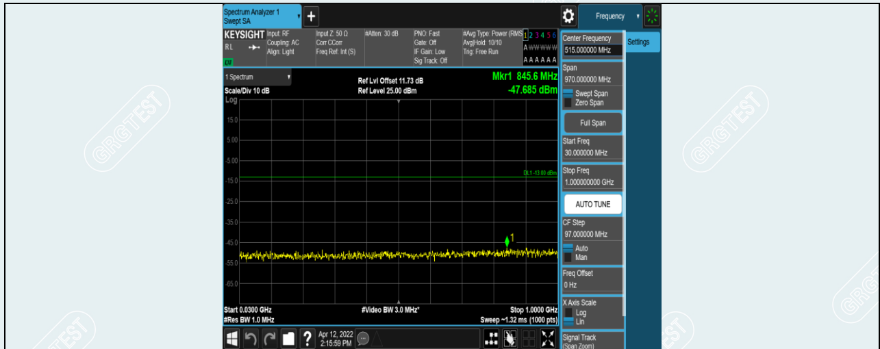
Band2-20MHz-QPSK-18700-1RB#0-Range1:30~1000MHz
