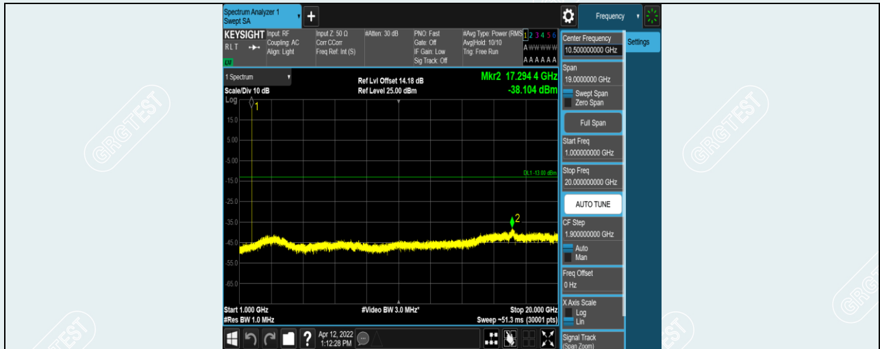
Band4-1.4MHz-QPSK-20175-1RB#0-Range2:1000~20000MHz
