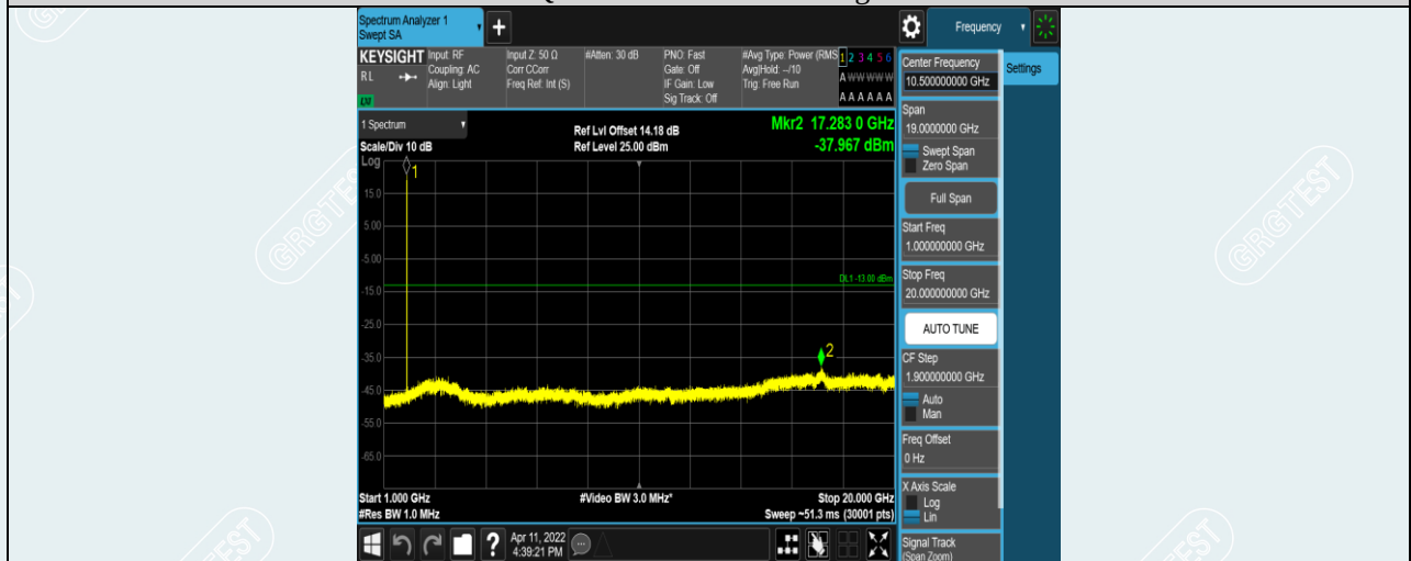
Band2-10MHz-QPSK-18650-1RB#0-Range2:1000~20000MHz
