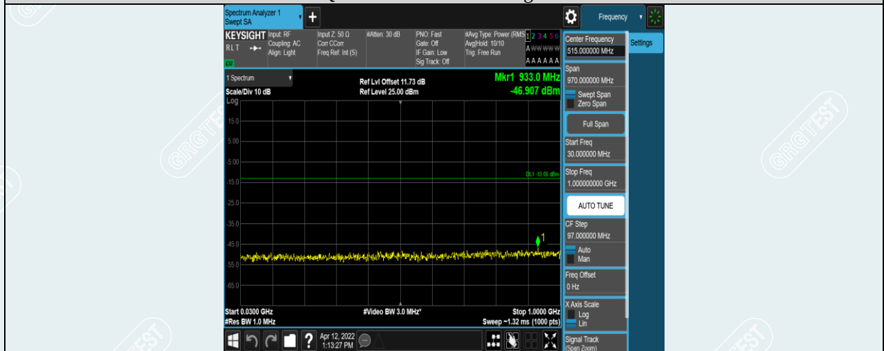
Band4-1.4MHz-QPSK-20393-1RB#0-Range1:30~1000MHz
