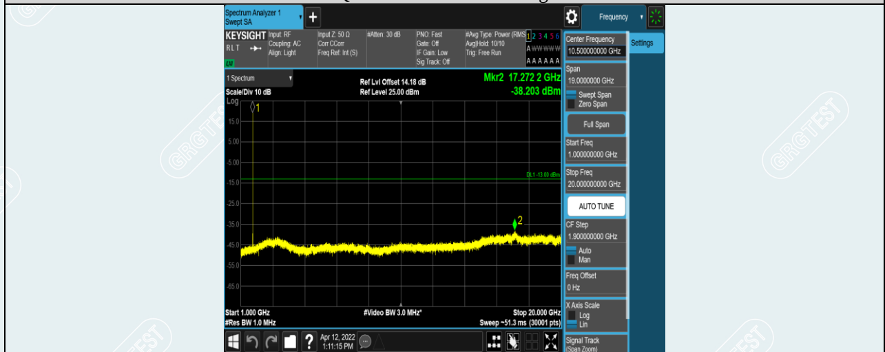
Band4-1.4MHz-QPSK-19957-1RB#0-Range2:1000~20000MHz
