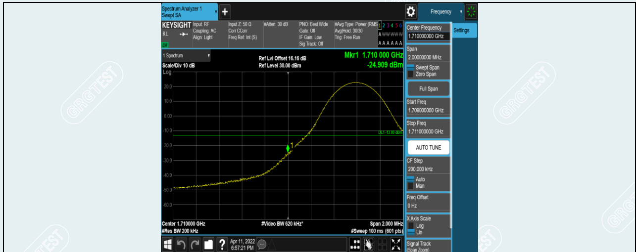
Band4-10MHz-QPSK-20000-1RB#0
