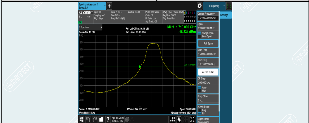
Band4-3MHz-QPSK-19965-1RB#0
