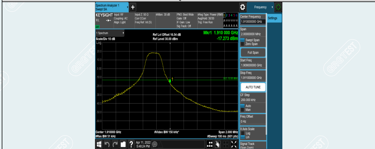
Band2-3MHz-QPSK-19185-1RB#14
