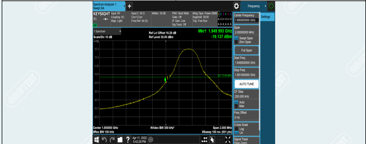
Band2-5MHz-16QAM-18625-1RB#0
