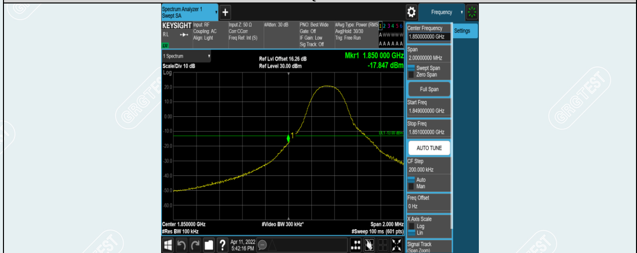
Band2-5MHz-QPSK-18625-1RB#0
