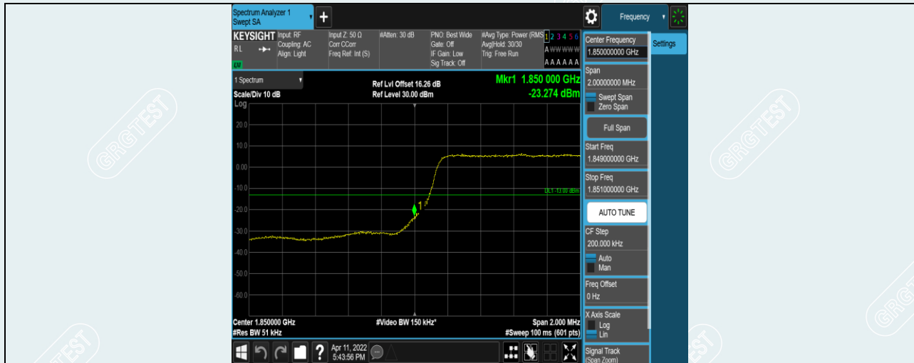
Band2-3MHz-QPSK-18615-15RB#0
