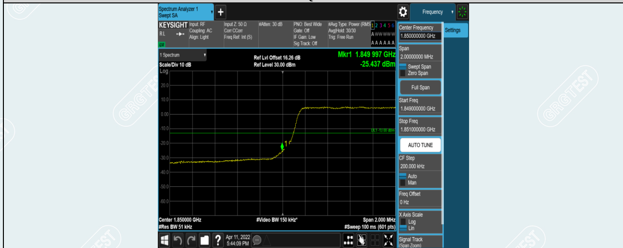
Band2-3MHz-16QAM-18615-15RB#0
