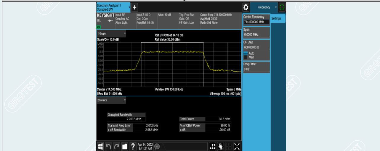
Band12-3MHz-QPSK-23165-15RB#0
