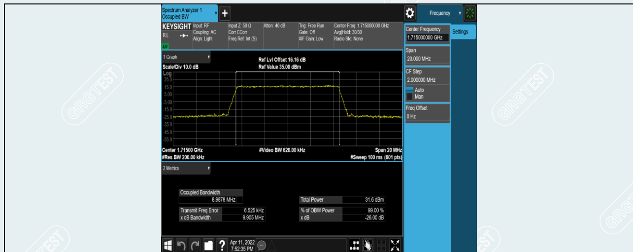
Band4-10MHz-QPSK-20000-50RB#0
