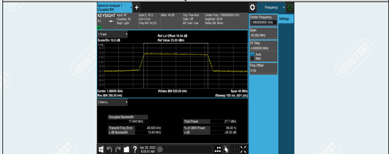
Band2-20MHz-QPSK-18900-100RB#0
