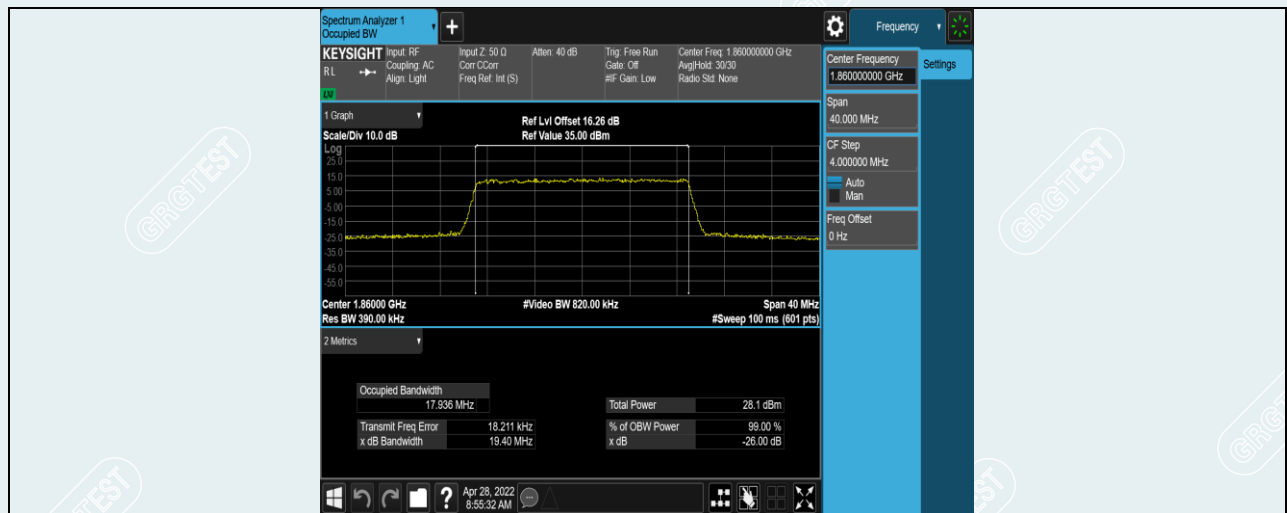
Band2-20MHz-QPSK-18700-100RB#0
