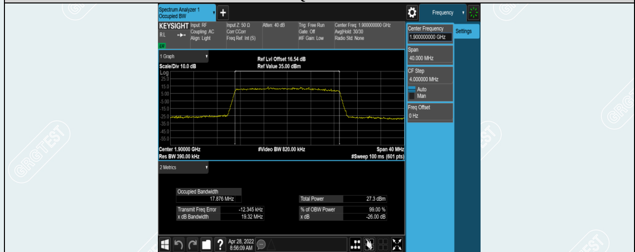
Band2-20MHz-QPSK-19100-100RB#0
