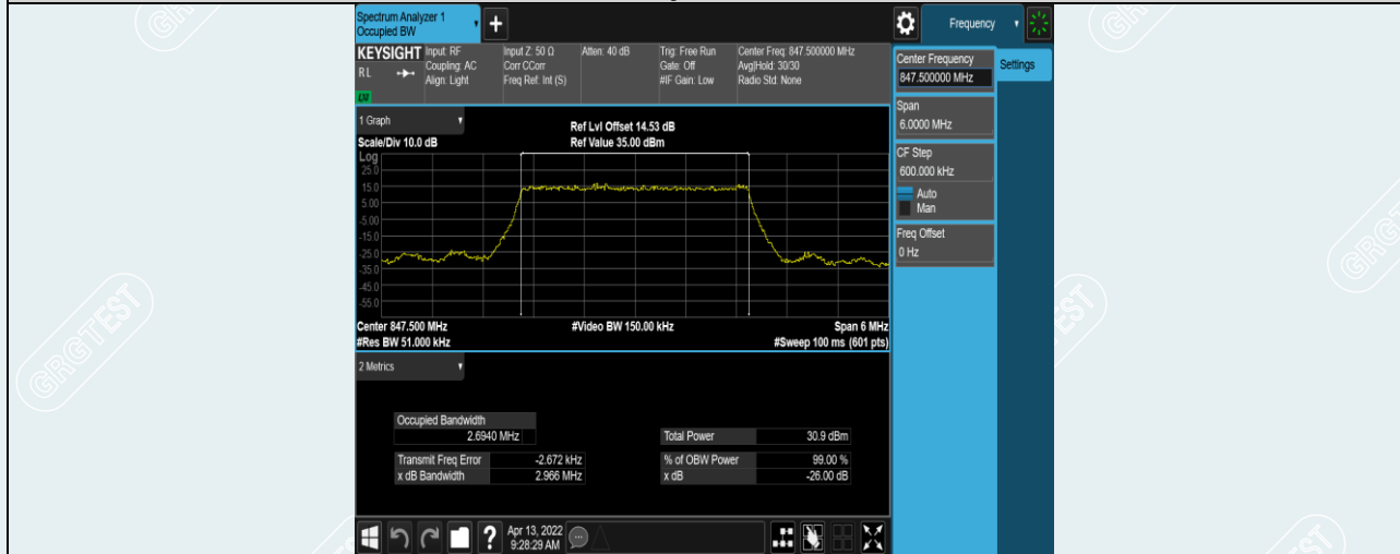
Band5-3MHz-QPSK-20635-15RB#0
