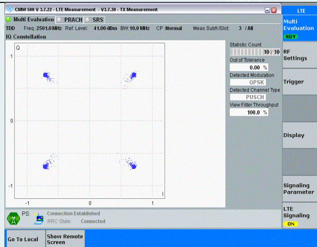
Band41-10MHz-QPSK-39700-50RB#0
