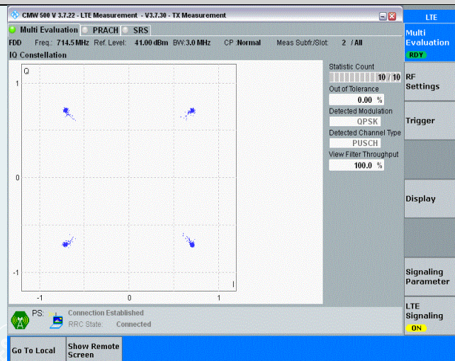
Band12-3MHz-QPSK-23165-15RB#0
