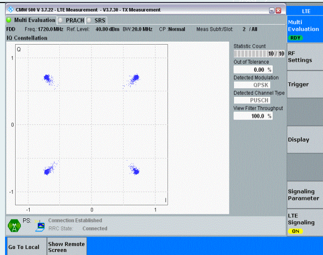
Band4-20MHz-QPSK-20050-100RB#0
