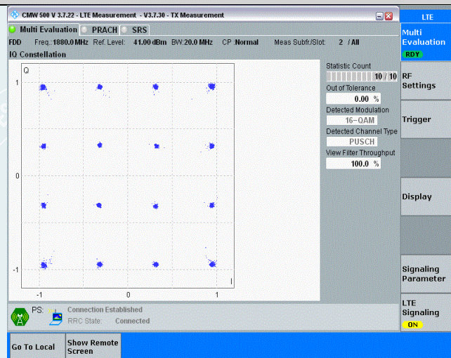
Band2-20MHz-16QAM-18900-100RB#0
