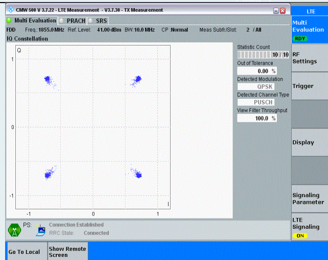
Band2-10MHz-QPSK-18650-50RB#0
