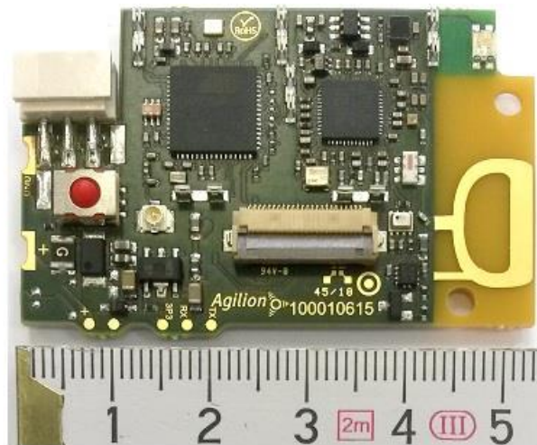
PCB top
