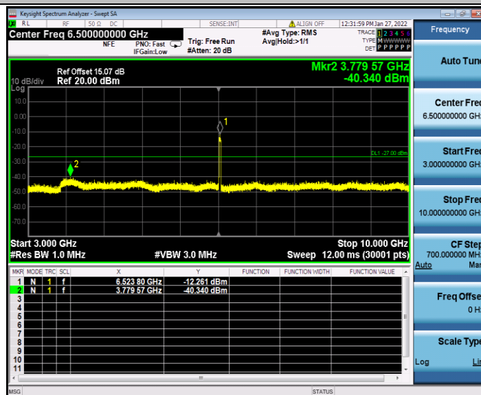
11AX40MIMO_Ant2_6525_3000~10000
