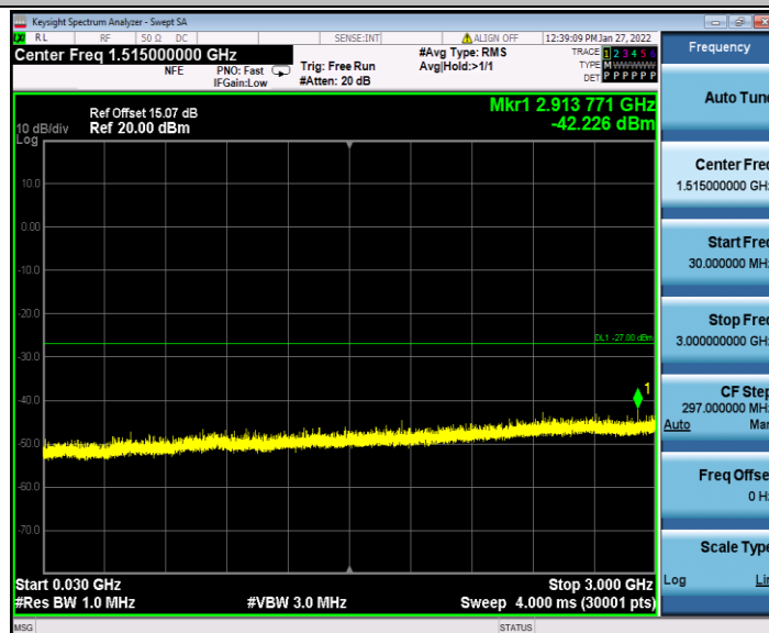
11AX40MIMO_Ant2_6565_30~3000
