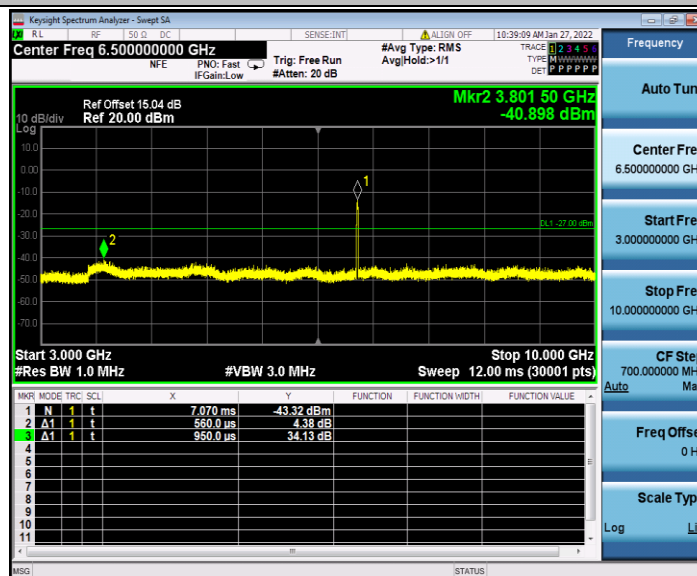
11AX20MIMO_Ant1_6995_3000~10000
