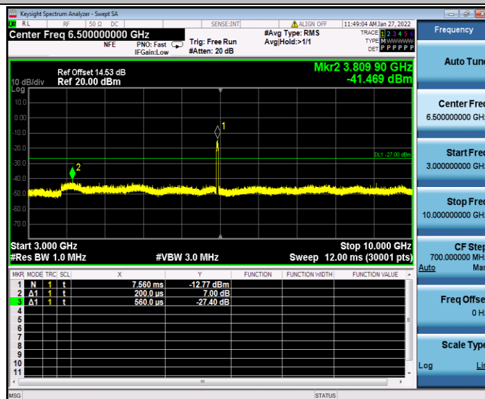
11AX40MIMO_Ant1_6445_3000~10000
