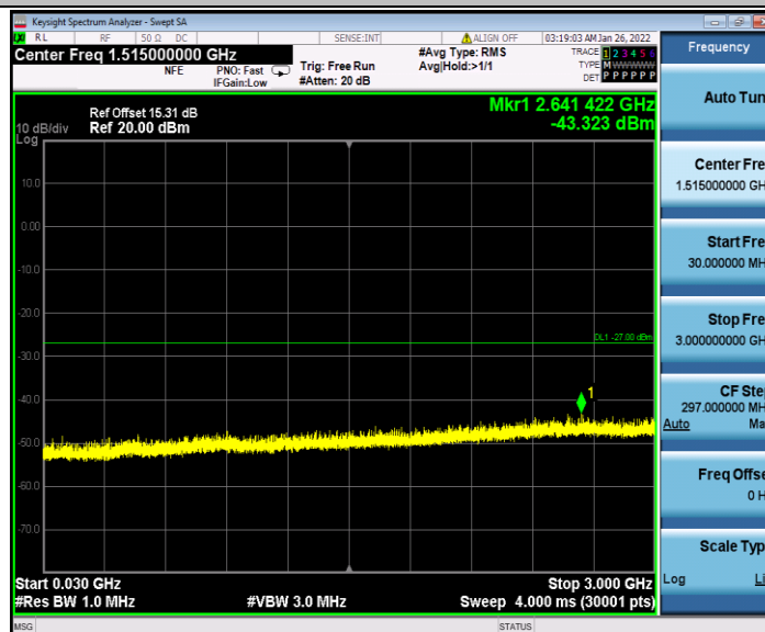
11N40MIMO_Ant2_7085_30~3000
