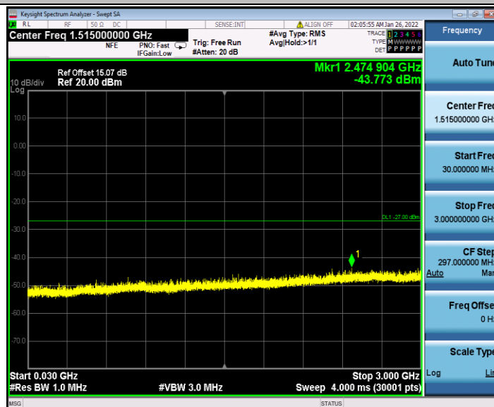
11N40MIMO_Ant2_6685_30~3000
