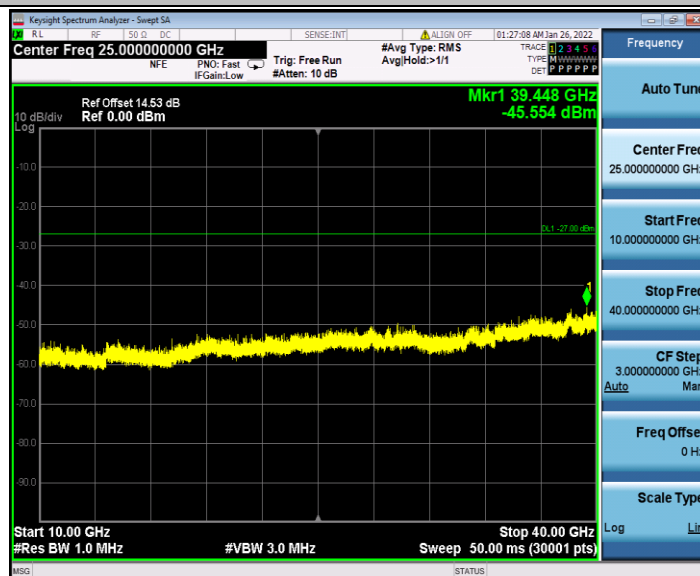
11N40MIMO_Ant1_6445_10000~40000
