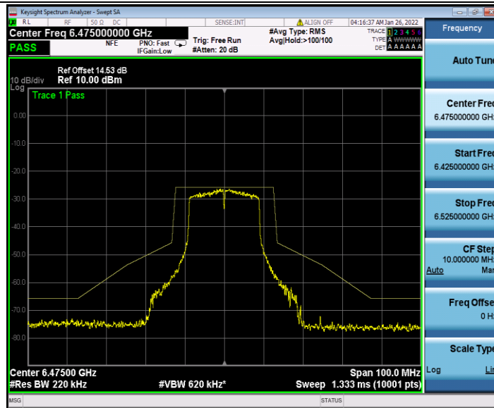
11AC20MIMO_Ant2_6475
