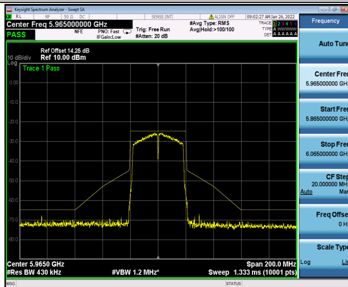
11AC40MIMO_Ant2_5965
