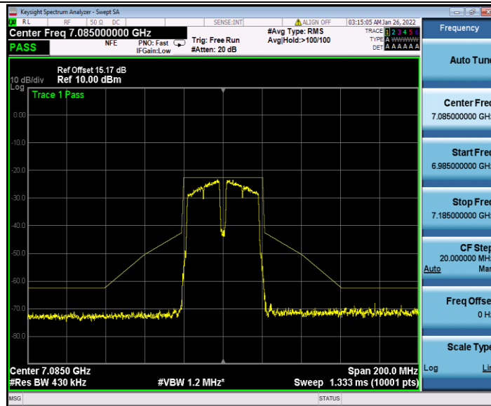
11N40MIMO_Ant2_7085
