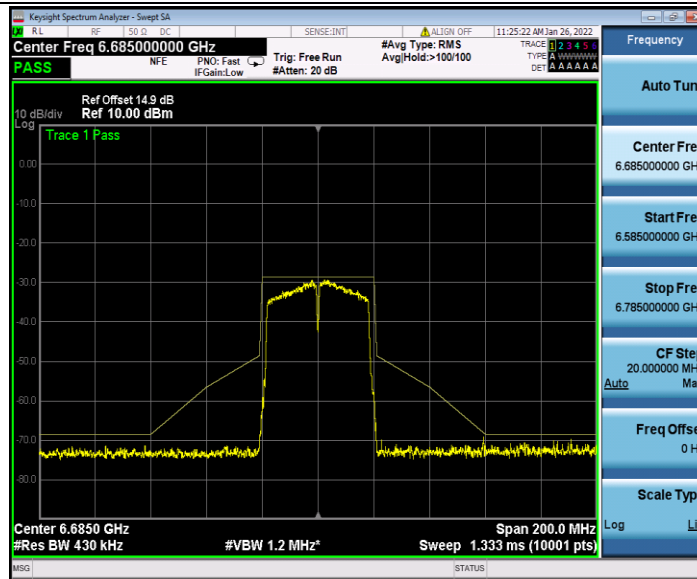
11AC40MIMO_Ant2_6685
