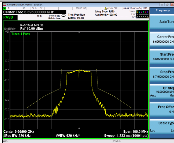
11AC20MIMO_Ant2_6695
