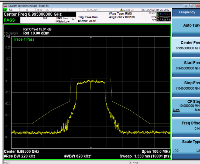
11AC20MIMO_Ant1_6995
