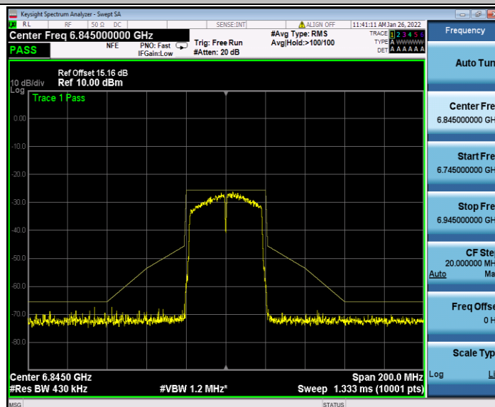
11AC40MIMO_Ant1_6845
