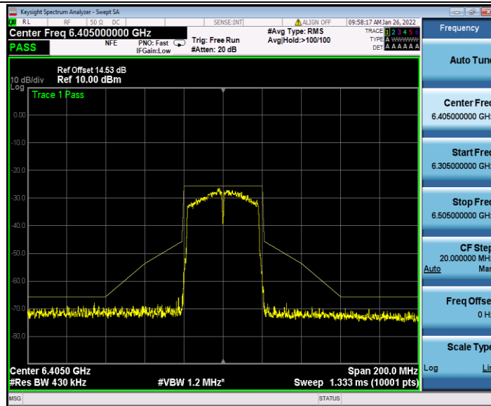
11AC40MIMO_Ant2_6405
