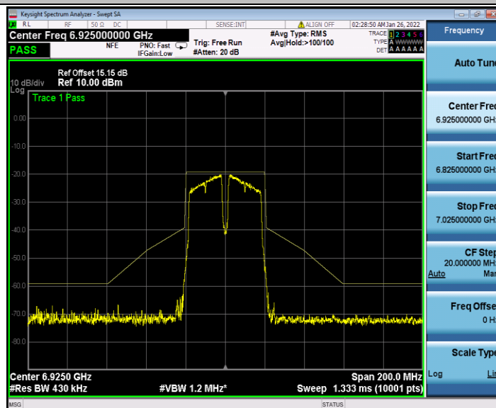
11N40MIMO_Ant2_6925
