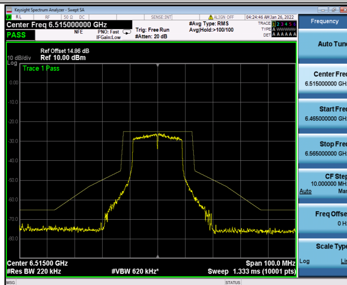
11AC20MIMO_Ant1_6515
