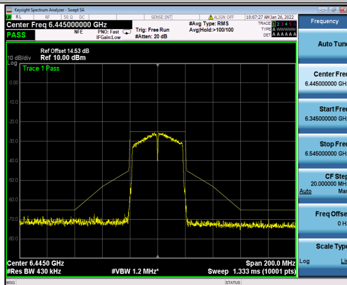
11AC40MIMO_Ant1_6445
