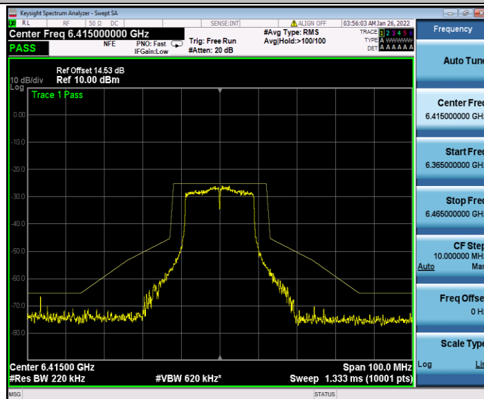
11AC20MIMO_Ant2_6415
