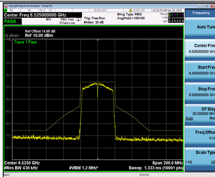
11AC40MIMO_Ant2_6525
