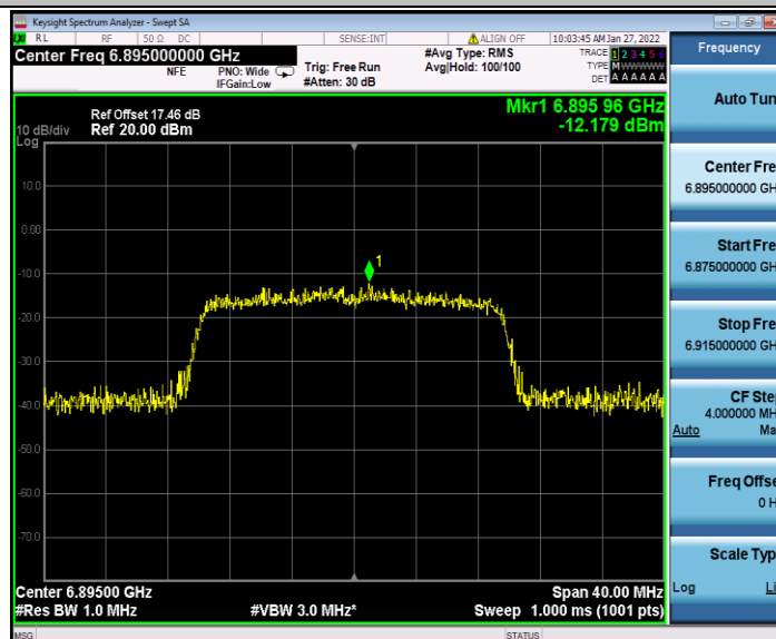
11AX20MIMO_Ant1_6895
