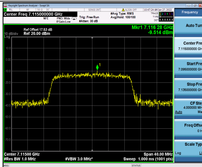
11AX20MIMO_Ant2_7115
