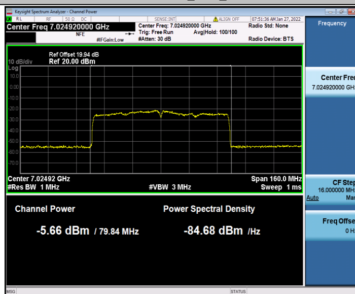
11AC80MIMO_Ant1_7025
