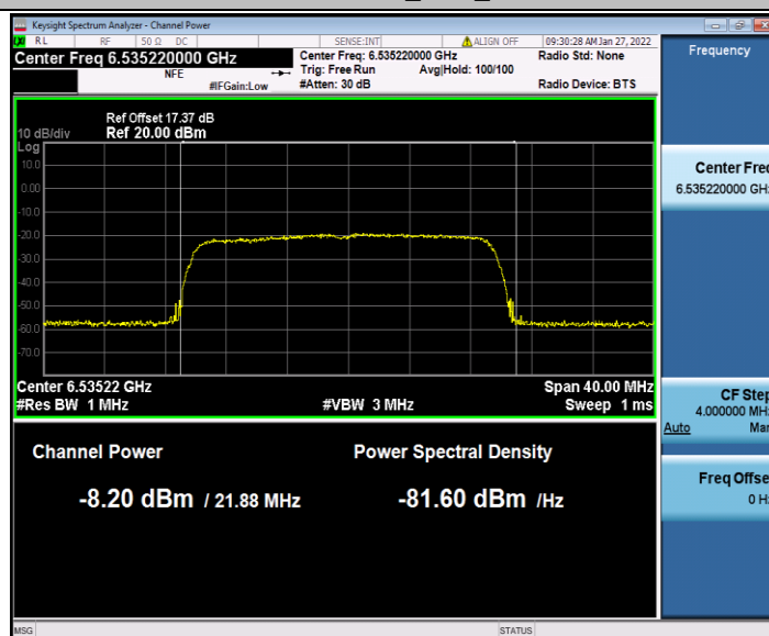
11AX20MIMO_Ant2_6535
