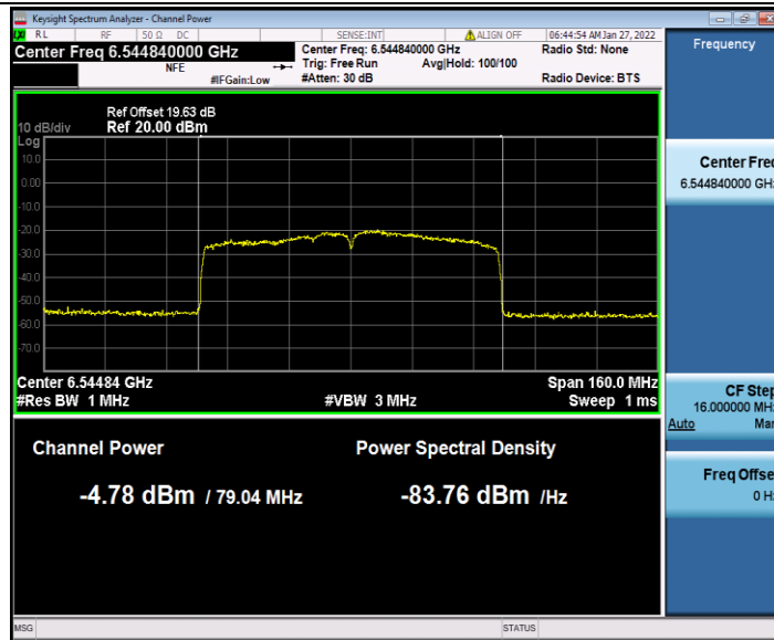
11AC80MIMO_Ant2_6545
