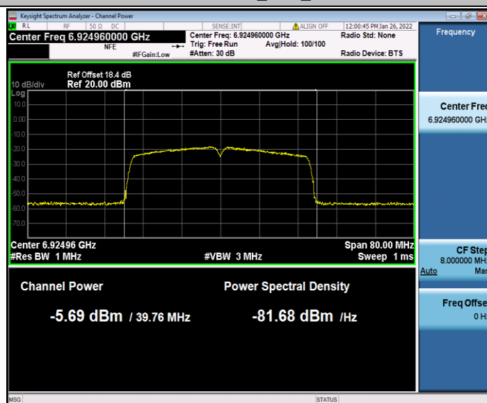
11AC40MIMO_Ant2_6925
