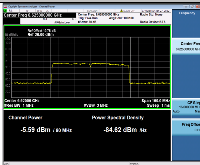
11AC80MIMO_Ant1_6625
