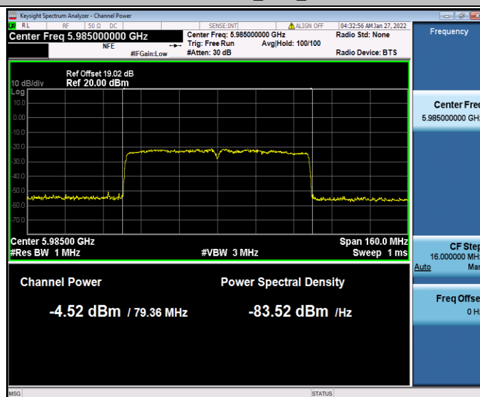
11AC80MIMO_Ant1_5985
