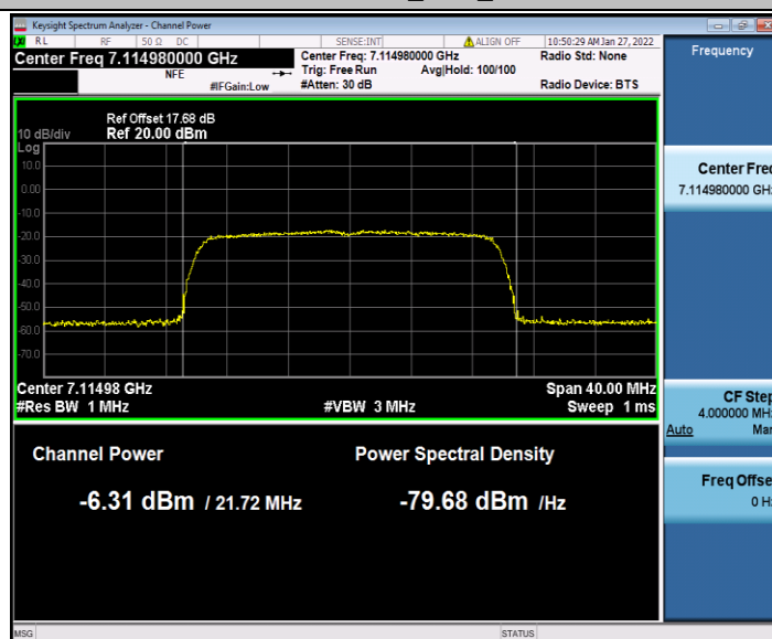
11AX20MIMO_Ant2_7115
