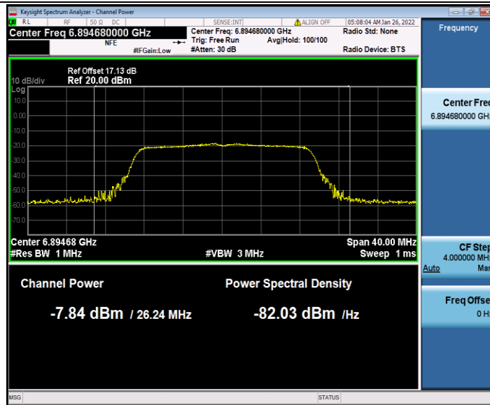
11AC20MIMO_Ant2_6895
