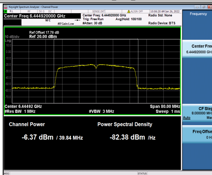
11AC40MIMO_Ant1_6445
