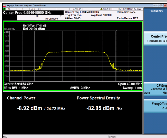
11AC20MIMO_Ant1_6995
