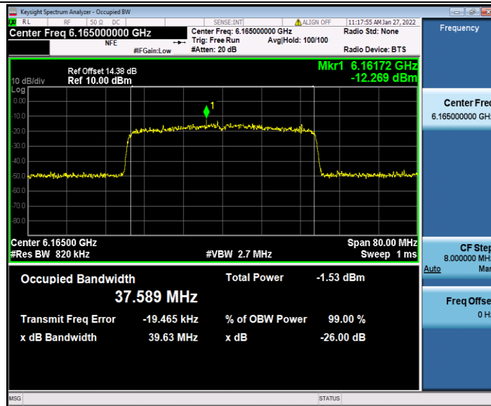
11AX40MIMO_Ant2_6165
