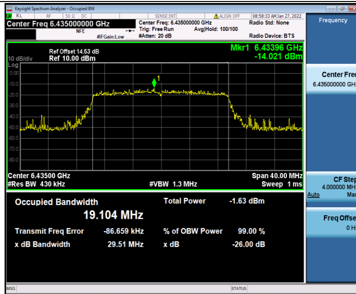
11AX20MIMO_Ant2_6435
