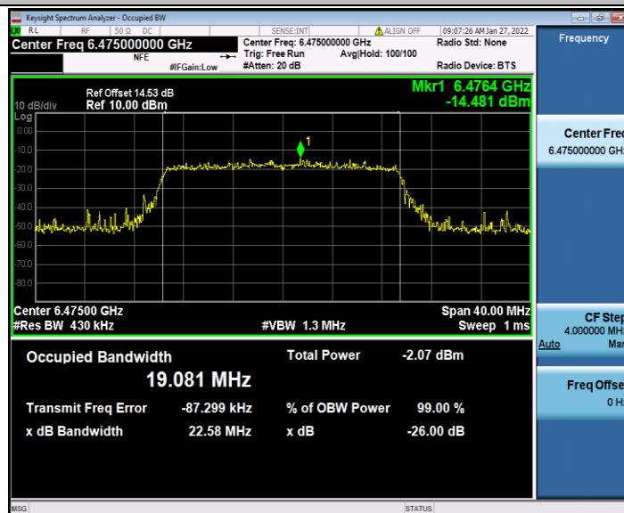
11AX20MIMO_Ant1_6475
