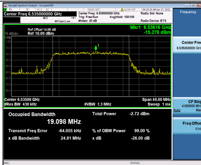
11AX20MIMO_Ant2_6535
