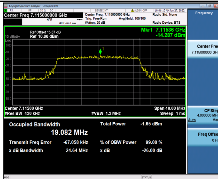
11AX20MIMO_Ant2_7115
