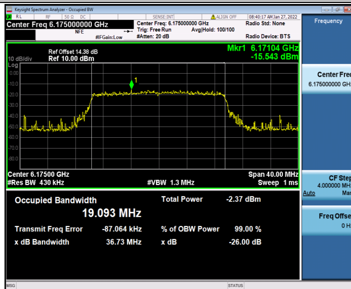
11AX20MIMO_Ant2_6175
