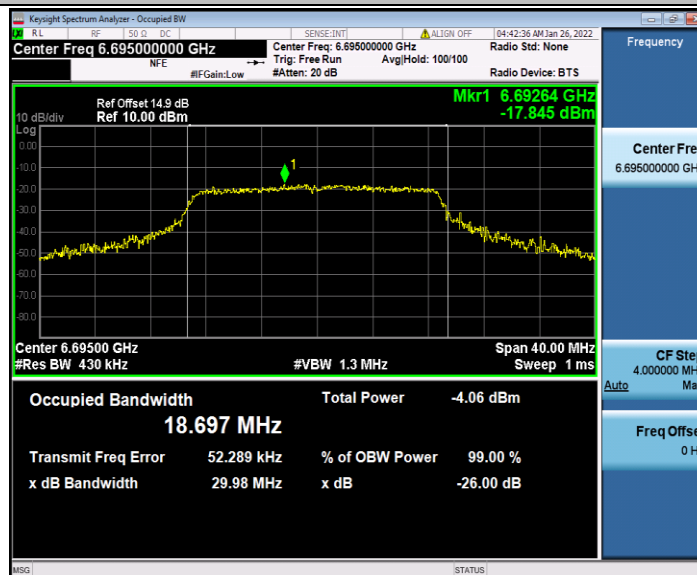
11AC20MIMO_Ant2_6695
