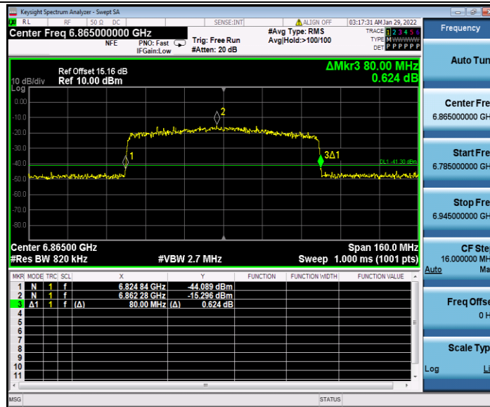
11AX80MIMO_Ant2_6865
