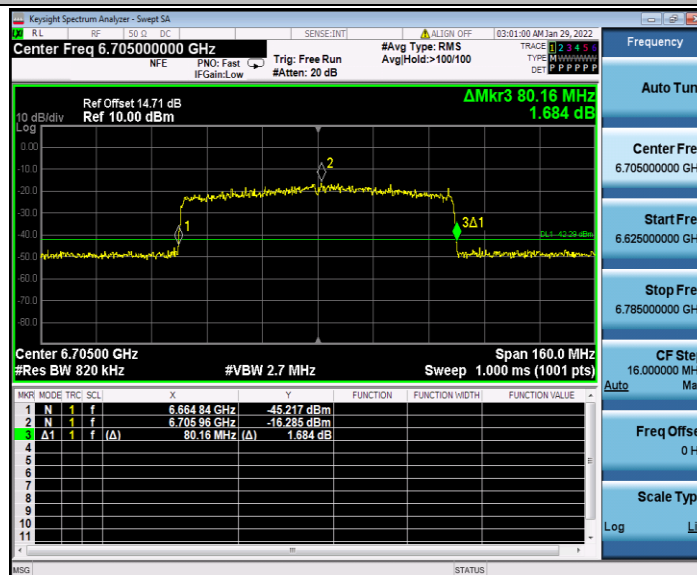
11AX80MIMO_Ant2_6705
