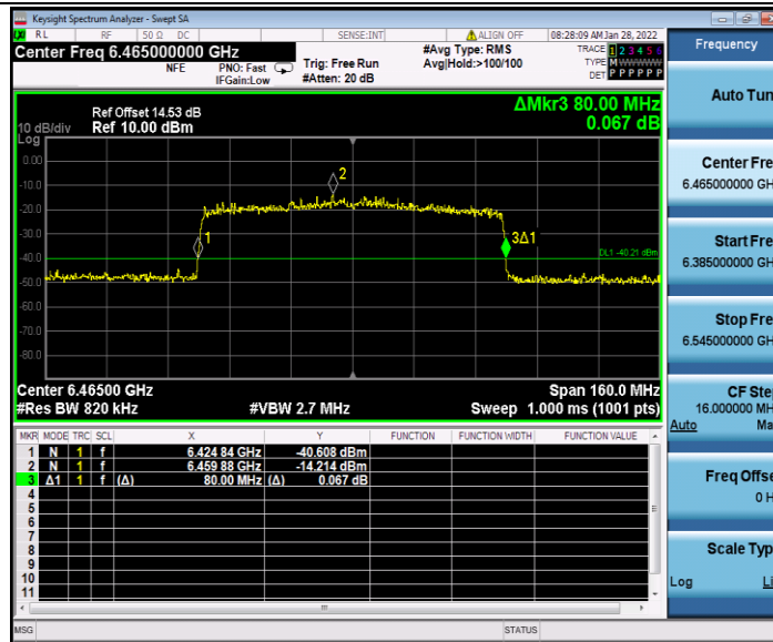
11AX80MIMO_Ant2_6465
