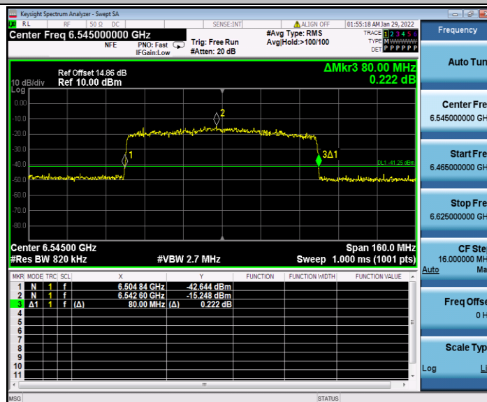
11AX80MIMO_Ant1_6545
