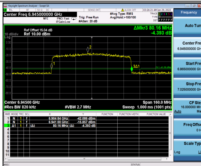
11AX80MIMO_Ant1_6945
