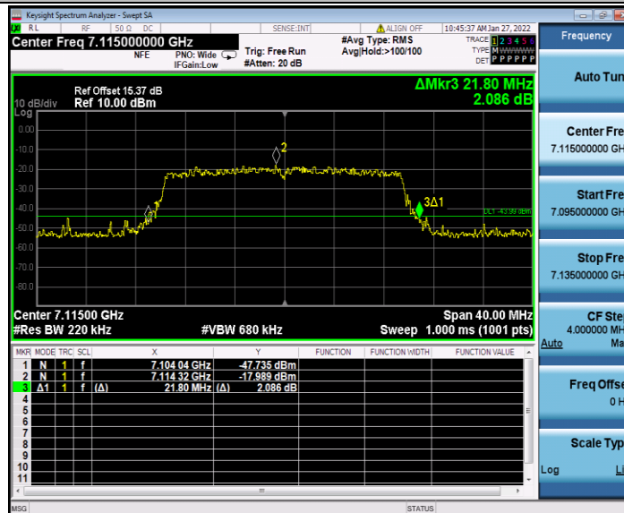
11AX20MIMO_Ant2_7115
