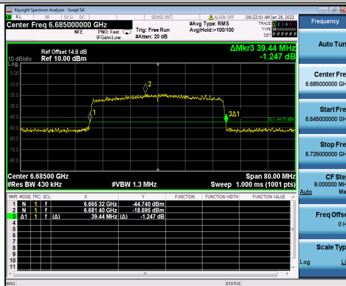
11AX40MIMO_Ant1_6685
