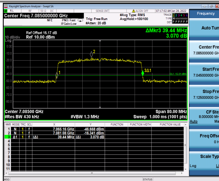
11AX40MIMO_Ant1_7085
