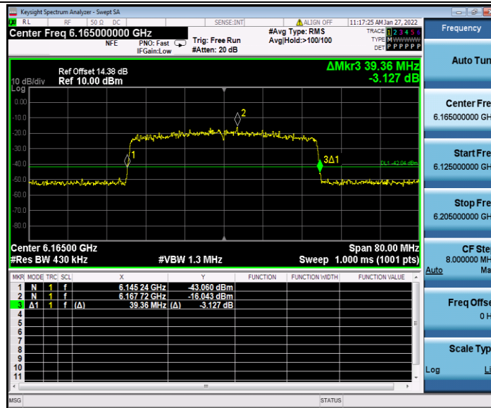
11AX40MIMO_Ant2_6165
