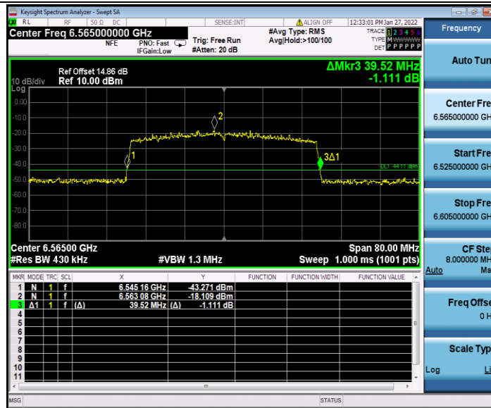
11AX40MIMO_Ant2_6565
