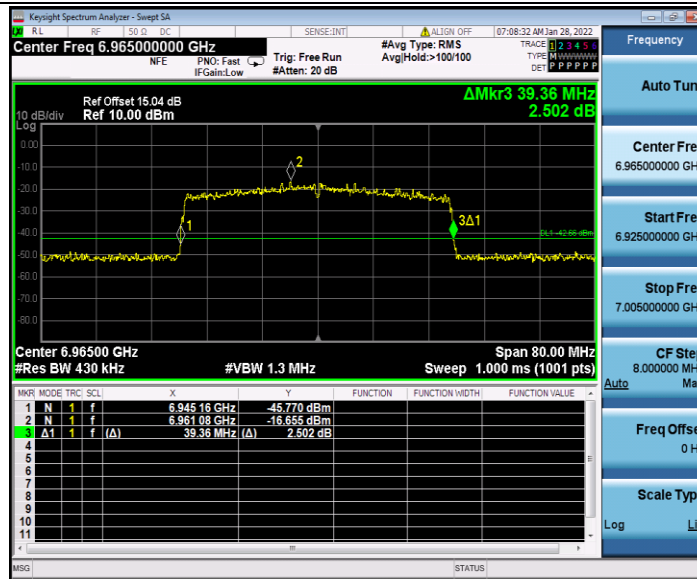
11AX40MIMO_Ant2_6965
