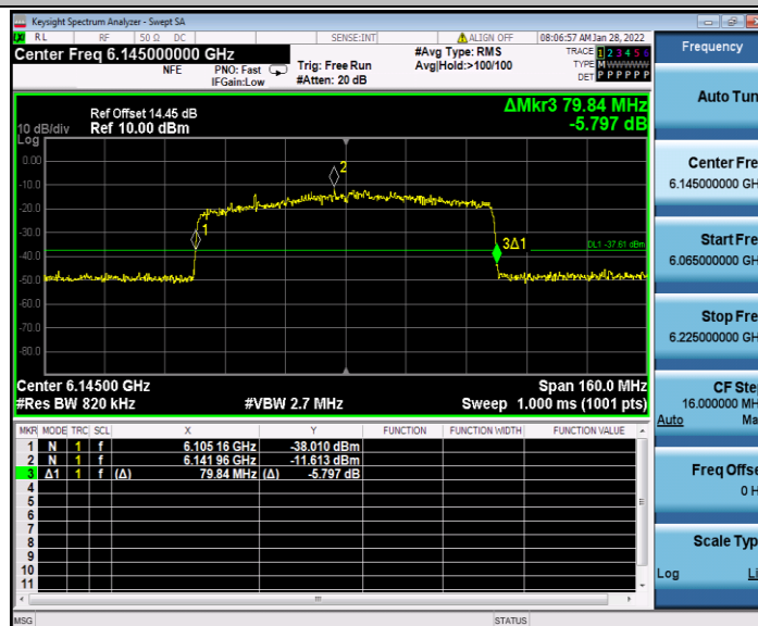
11AX80MIMO_Ant2_6145
