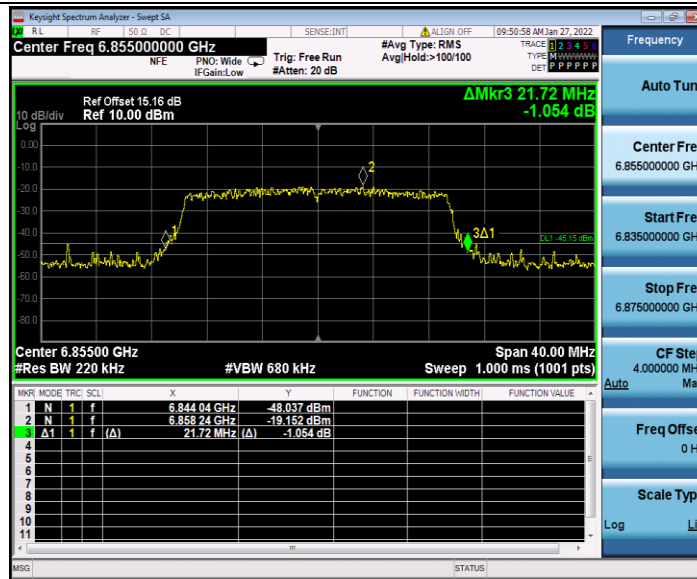
11AX20MIMO_Ant2_6855
