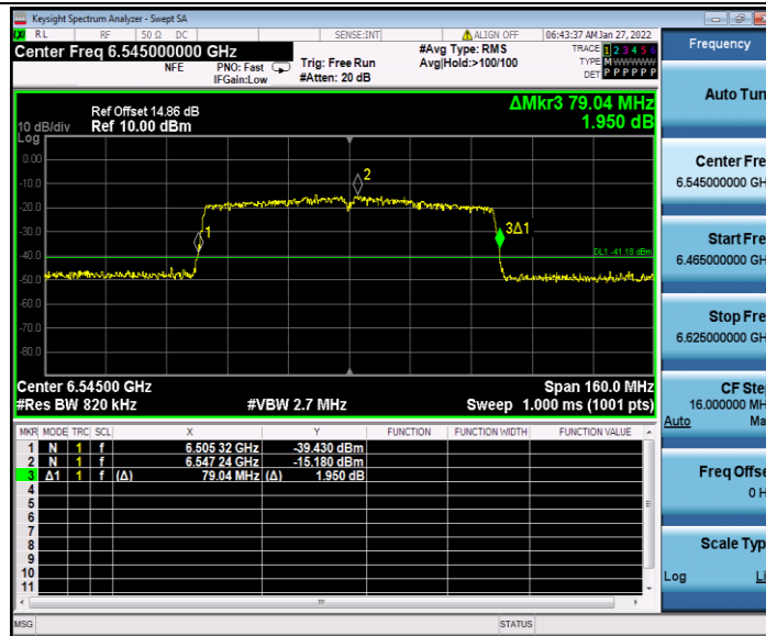
11AC80MIMO_Ant2_6545
