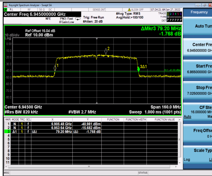
11AC80MIMO_Ant2_6945
