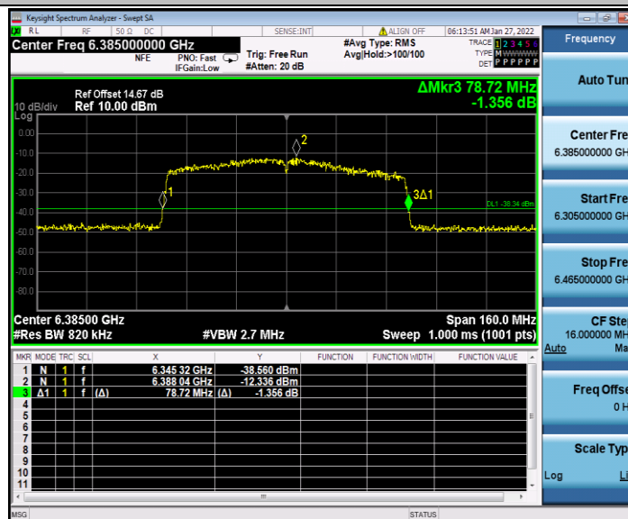
11AC80MIMO_Ant2_6385
