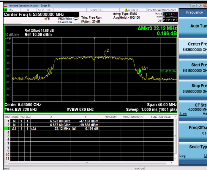
11AX20MIMO_Ant2_6535
