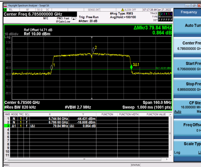
11AC80MIMO_Ant2_6785
