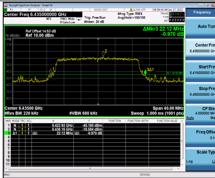
11AX20MIMO_Ant2_6435
