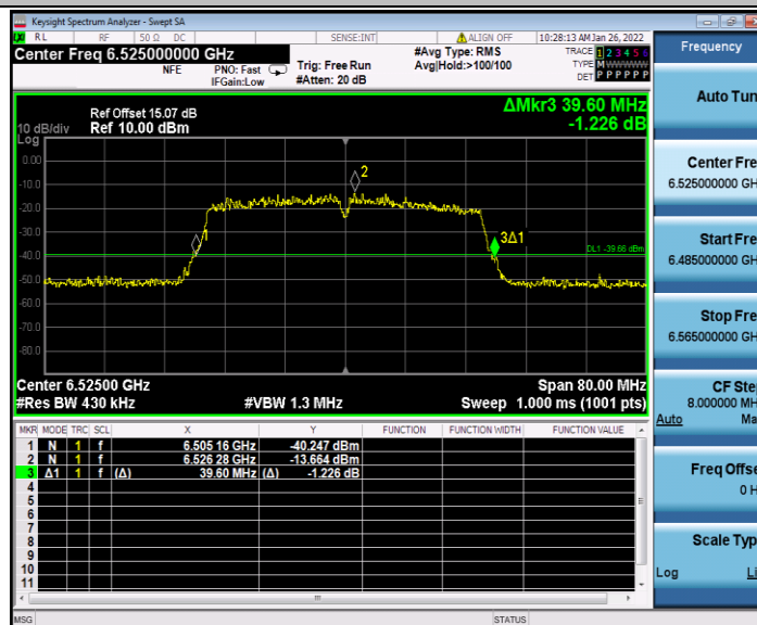
11AC40MIMO_Ant2_6525
