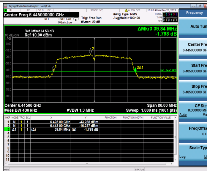
11AC40MIMO_Ant1_6445
