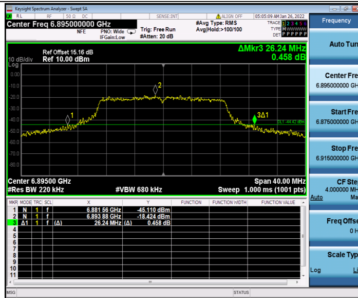
11AC20MIMO_Ant2_6895
