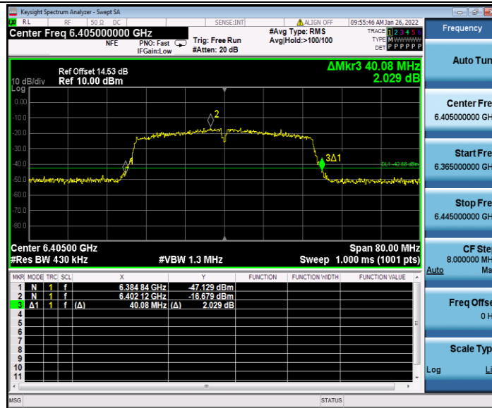
11AC40MIMO_Ant2_6405
